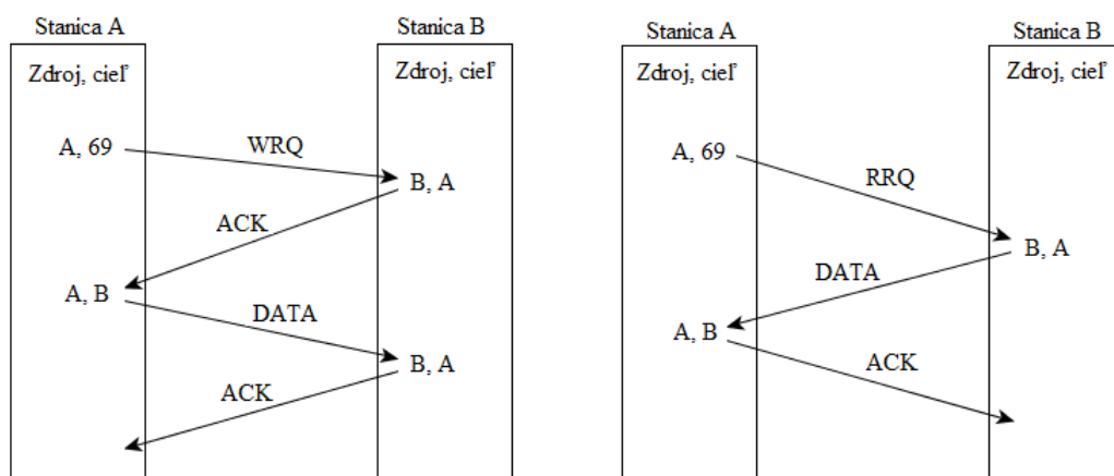
Obr. 4.1: Vytvorenie spojenia pri požiadavke na zápis a na čítanie.
