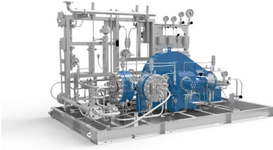
Obr. 7 Vodíkový kompresor [12]
