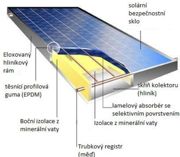
Obr. 6 Řez plochým kolektorem [27]
