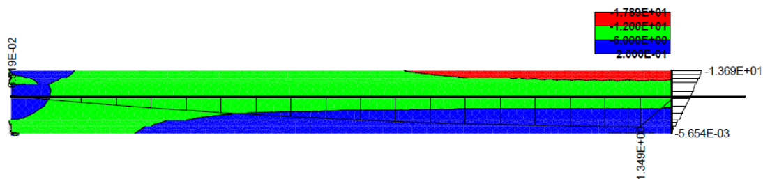
Obrázek 3.26: Priebeh hlavných normálových napätí Stress-Sigma xx v MPa + priebeh ohybových momentov v MNm, pre model s rozptýlenou šmykovou výstužou
