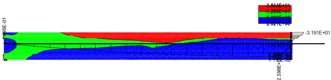
Obrázek 3.31: Priebek hlavných normálových napätí Stress-Sigma xx v MPa + priebek ohybových momentov v MNm, pre model bez šmykovej výstuže
