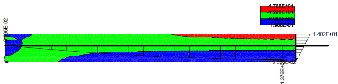
Obrázek 3.27: Priebch hlavných normálových napätí Stress-Sigma xx v MPa + priebch ohybových momentov v MNm, pre model s diskretnou šmykovou výstužou
