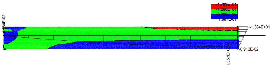
Obrázek 3.25: Priebeh hlavných normálových napätí Stress-Sigma xx v MPa + priebeh ohybových momentov v MNm, pre model bez šmykovej výstuže
