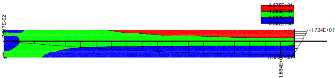
Obrázek 3.29: Priebch hlavných normálových napätí Stress-Sigma xx v MPa + priebch ohybových momentov v MNm, pre model s rozptýlenou šmykovou výstužou
