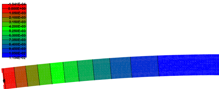
Obrázek 3.43: Vzopätie nosníka v násobku deformácie 50x pre model s diskretnou šmykovou výstužou
