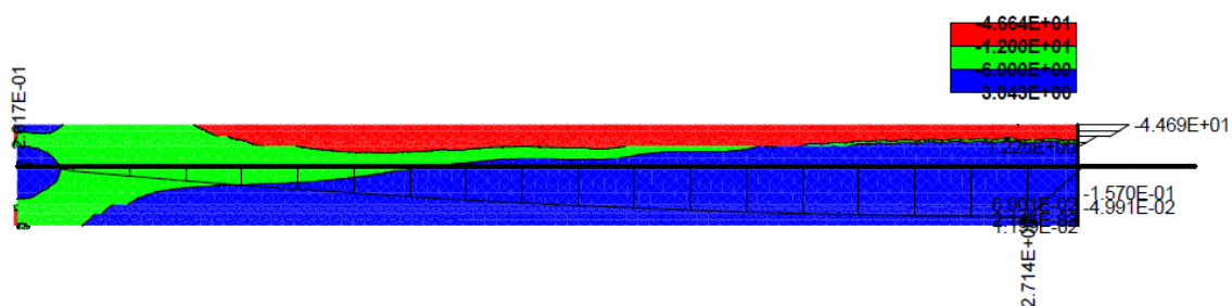
Obrázek 3.33: Priebeh hlavných normálových napätí Stress-Sigma xx v MPa + priebeh ohybových momentov v MNm, pre model s diskrétnou šmykovou výstužou
