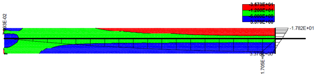
Obrázek 3.30: Priebek hlavných normálových napätí Stress-Sigma xx v MPa + priebek ohybových momentov v MNm, pre model s diskretnou šmykovou výstužou
