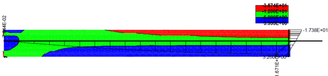
Obrázek 3.28: Priebch hlavných normálových napätí Stress-Sigma xx v MPa + priebch ohybových momentov v MNm, pre model bez šmykovej výstuže
