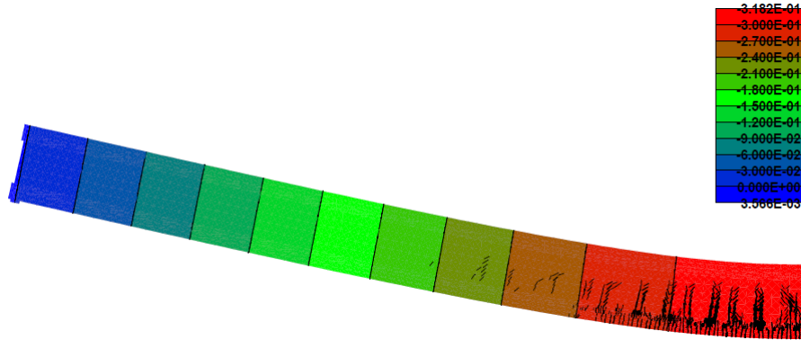
Obrázek 3.46: Pokles nosníka v násobku deformácie 5x pre model s diskrétnou šmykovou výstužou
