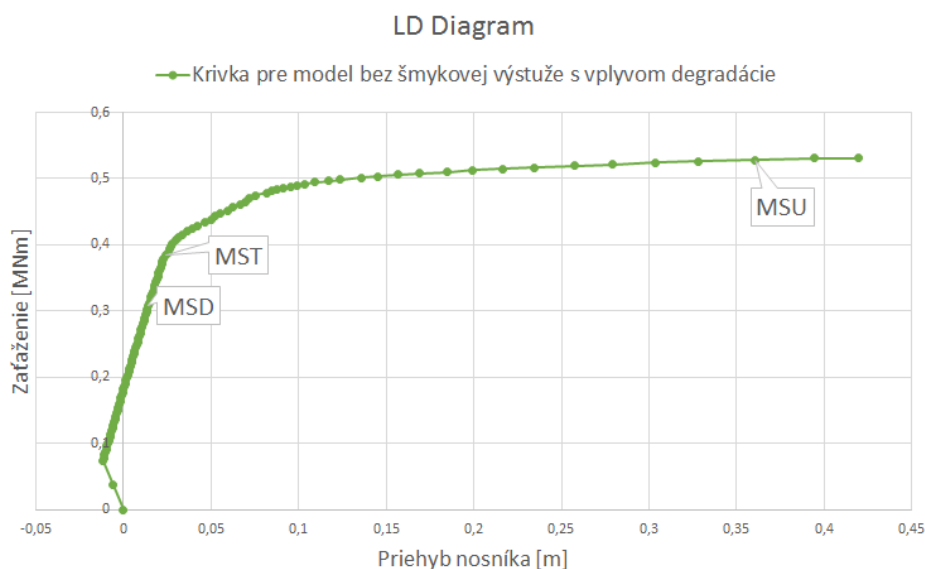
Obrázek 3.47: LD Diagram zafaženie–priehyb pre model bez šmykovej výstuže
