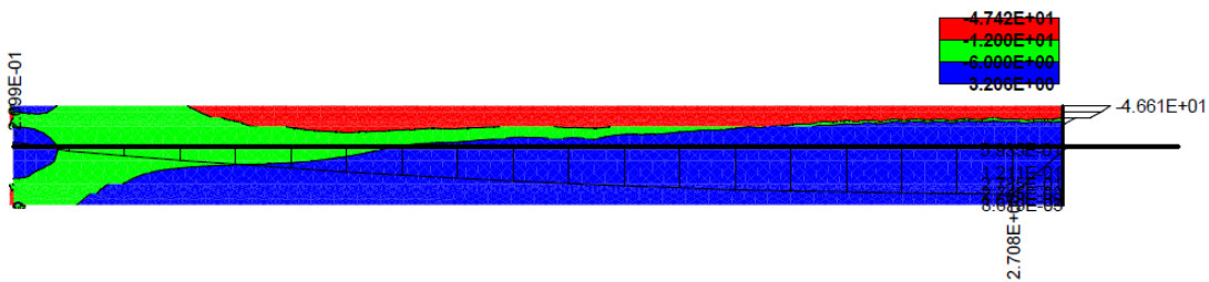
Obrázek 3.32: Priebek hlavných normálových napätí Stress-Sigma xx v MPa + priebek ohybových momentov v MNm, pre model s rozptýlenou šmykovou výstužou
