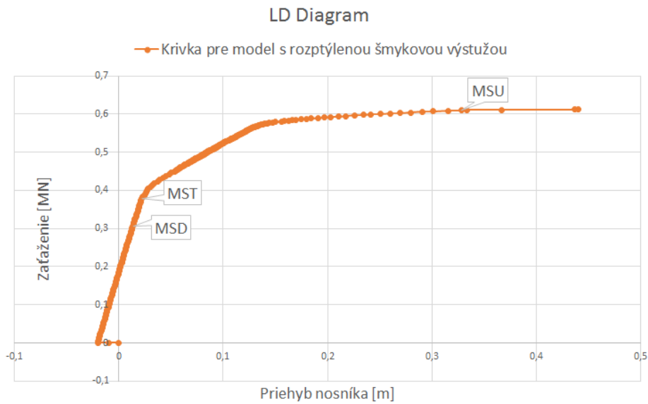
Obrázek 3.23: LD Diagram zaťaženie–priehyb pre model s rozptýlenou šmykovou výstužou
