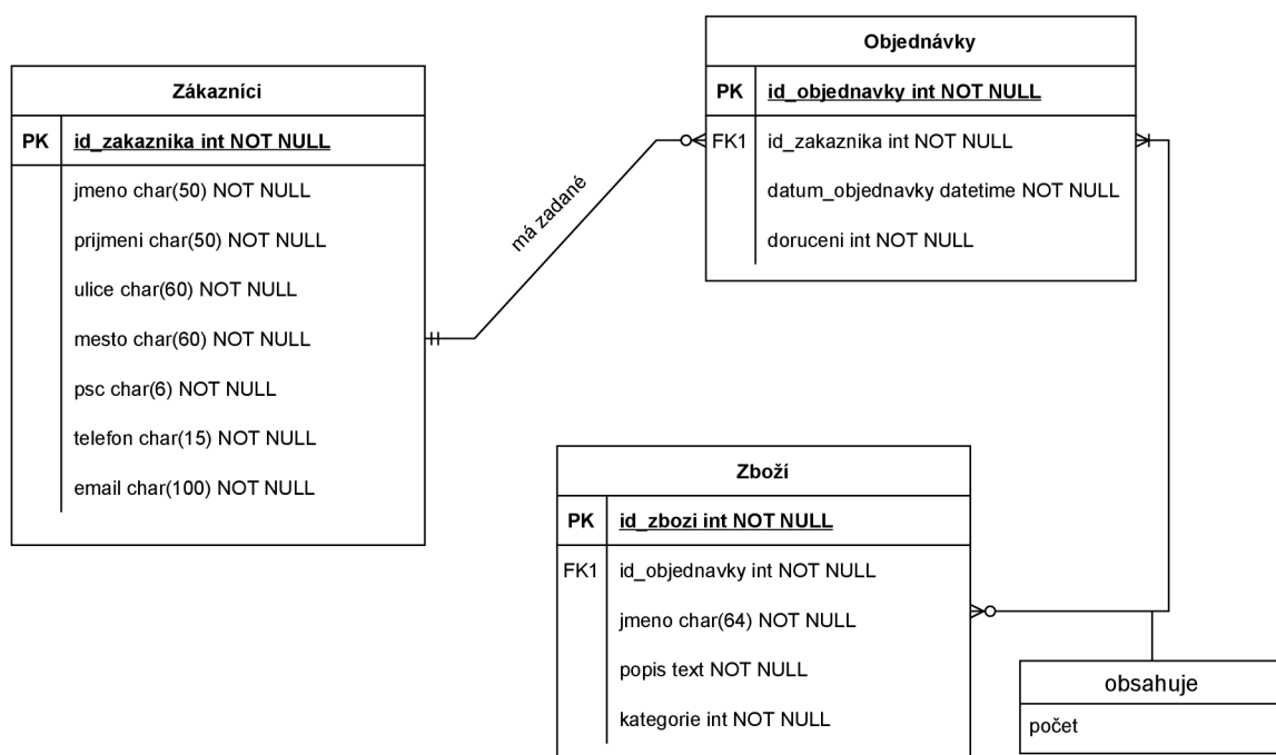
Obrázek 3.1: Příklad ER diagramu
