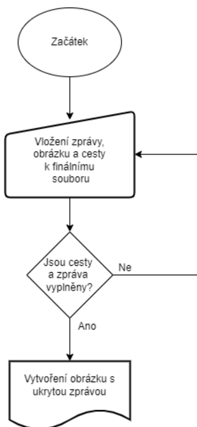
Obrázek 2.16: Vývojový diagram skrývání zprávy do souboru s formátem JPG.
