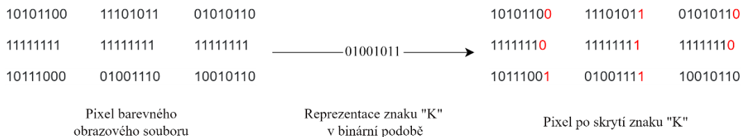
Obrázek 1.11: Vložení písmene „K“ do pixelu barevného obrazového souboru (vytvořen na základě [37]).
