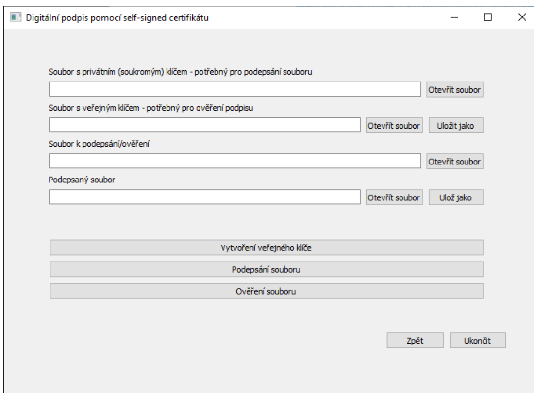
Obrázek 2.8: Okno digitálního podpisu za použití self-signed certifikátu.
