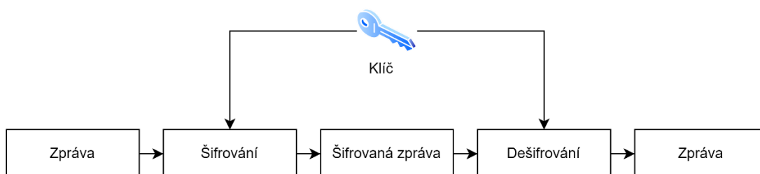
Obrázek 1.4: Symetrické šifrování.
