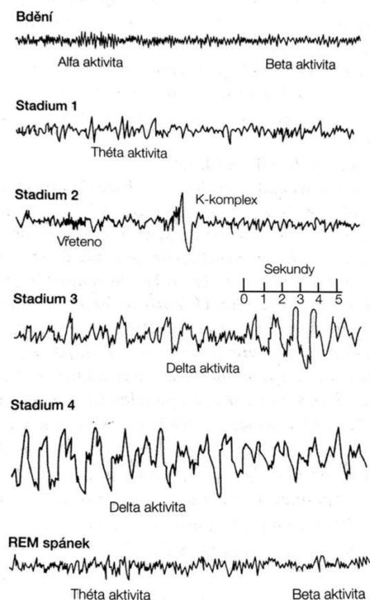
Obrázek 1: EEG záznam jednotlivých stadií spánku
