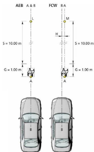
Obrázek 12: Schématický plán testu CPLA [32]
