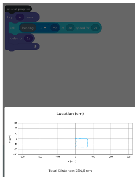
(b) Vykreslení čtverce s delay.
