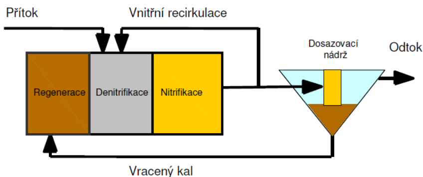
Obr. č. 3.1.3-8 Blokové schéma předřazené denitrifikace s regenerací kalu [26]
