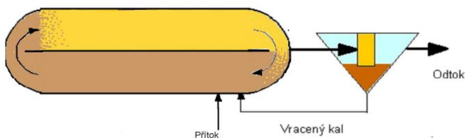
Obr. č. 3.1.3-10 Blokové schéma oběhové aktivace [26]
