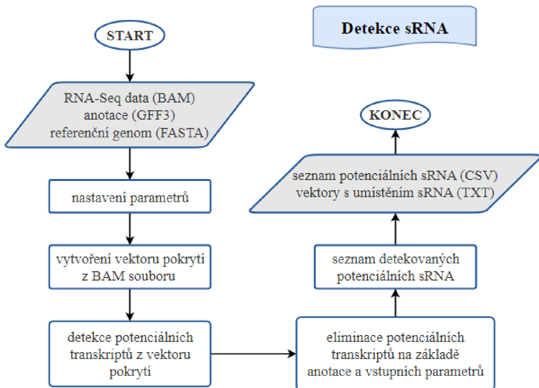
Obrázek 4.1 Zjednodušené schéma principu detekce nástroje SEARCHsRNA pro nalezení potenciálních sRNA.
