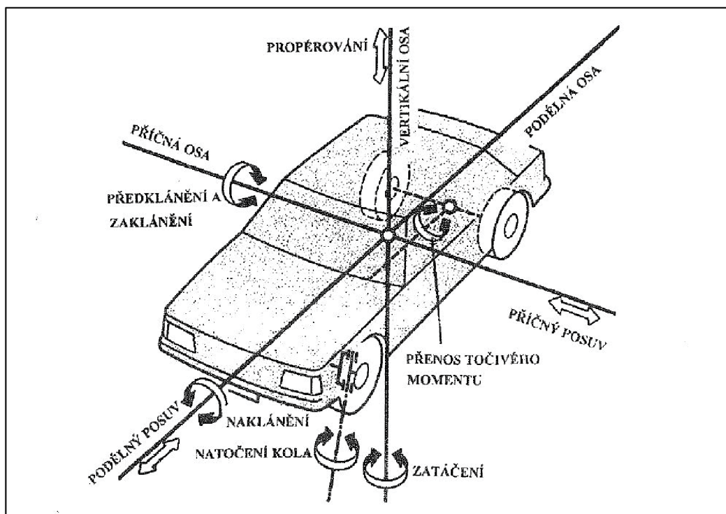
Obr. č. 25 - Pohyby, které vozidlo v závislosti na působících silách může vykonávat při jízdě [47]
