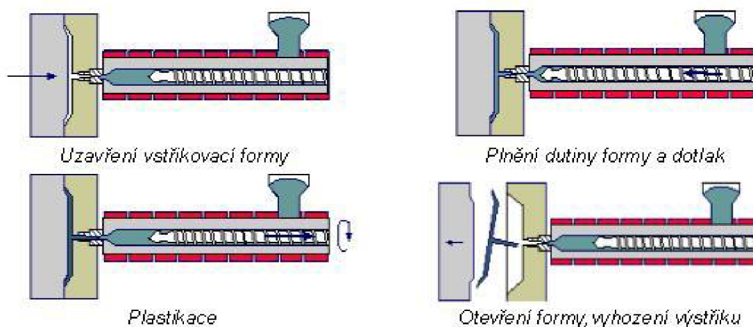
Obr. 1.5 Vstřikovací cyklus [5].
