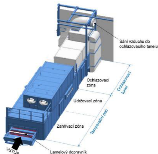
Obr. 1.11 Temperační pec [3].
