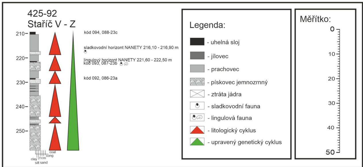
Obr. 10 Příklad vymezení litologického cyklu (červený trojúhelník) a upraveného genetického cyklu (zelený trojúhelník).
