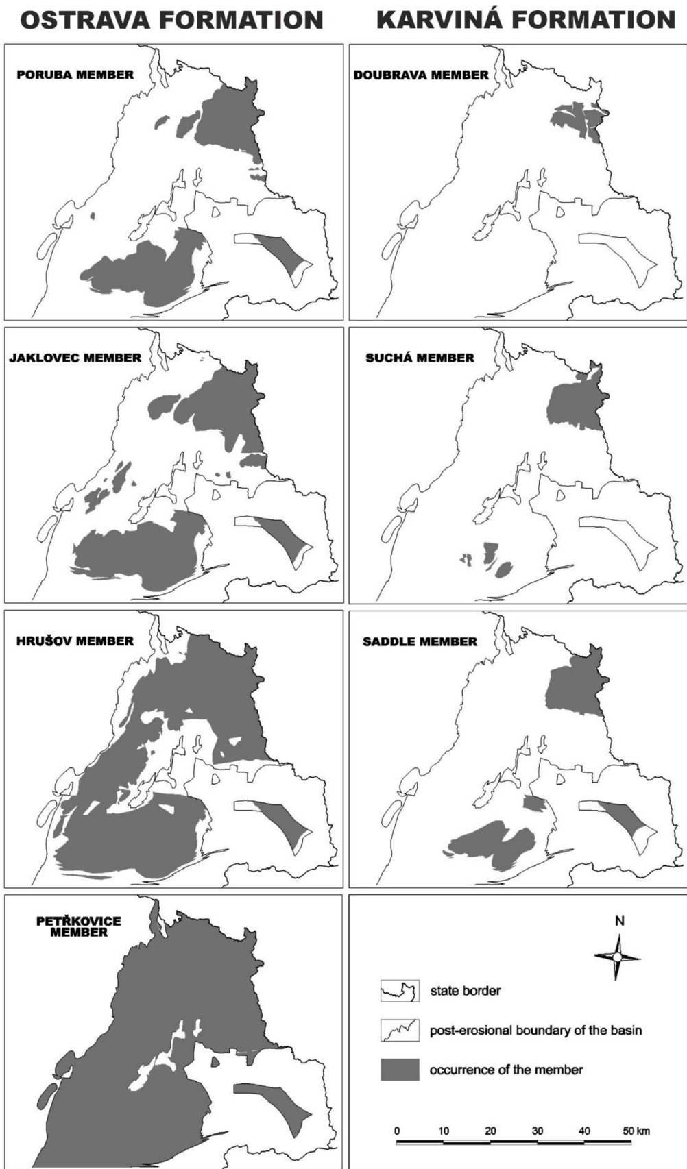
Obr. 3 Plošné rozšíření jednotlivých vrstev ostravského souvrství v ČHP (Kandarachevová et al. 2009).
