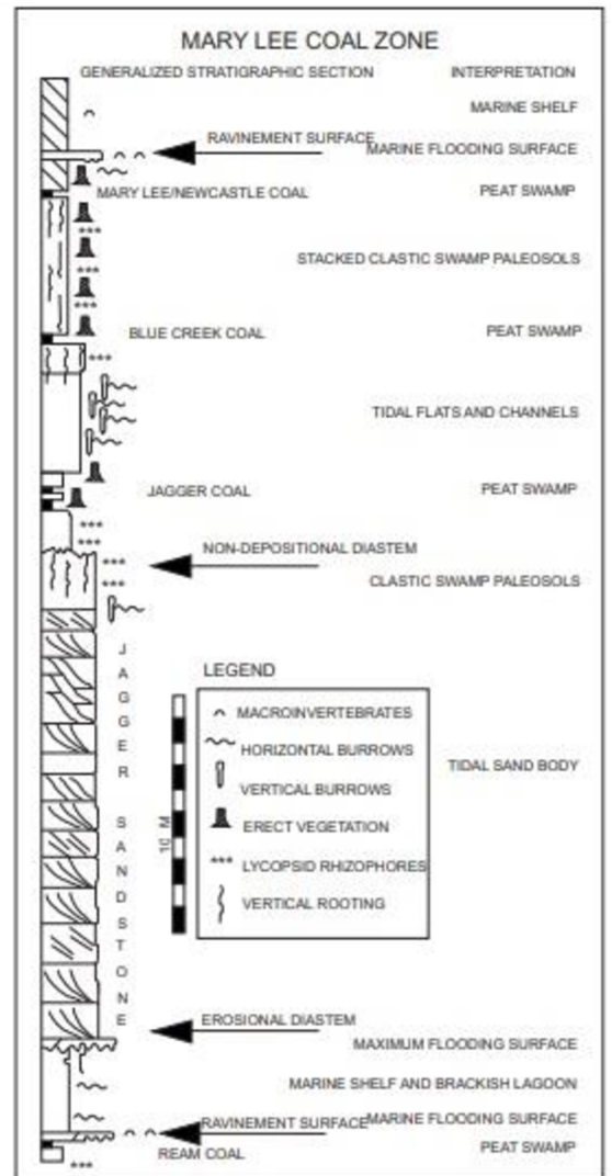
Obr. 7 Zobecněná stratigrafická sekvence pro zónu Mary Lee coal s interpretací jednotlivých depozičních prostředí (Gastaldo et al. 1993).
