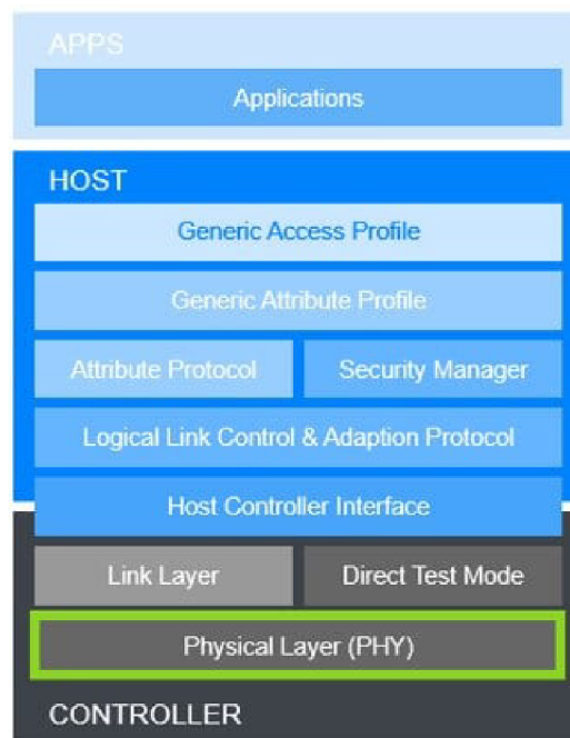
Obr. 3.1: Architektúra BLE[1]
