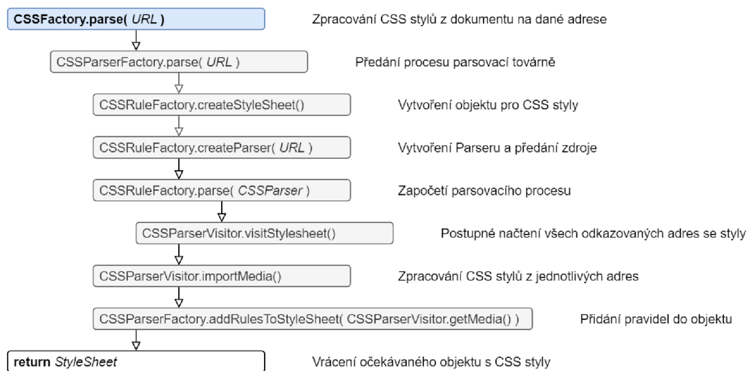
Obrázek 4.5: Diagram volání metody CSSFactory.parse()
