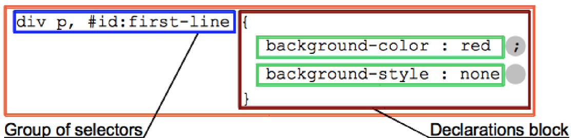
Obrázek 2.5: Ukázka syntaxe CSS pravidla [19]
