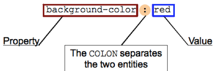
Obrázek 2.2: Ukázka syntaxe CSS deklarace [12]
