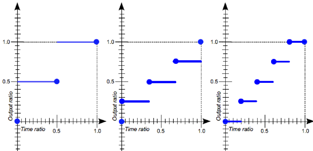
Obrázek 7.8: Průběh krokové funkce pro parametry (2, start ) [17], (3, jump-both ) [15] a (5, jump-none ) [16]
