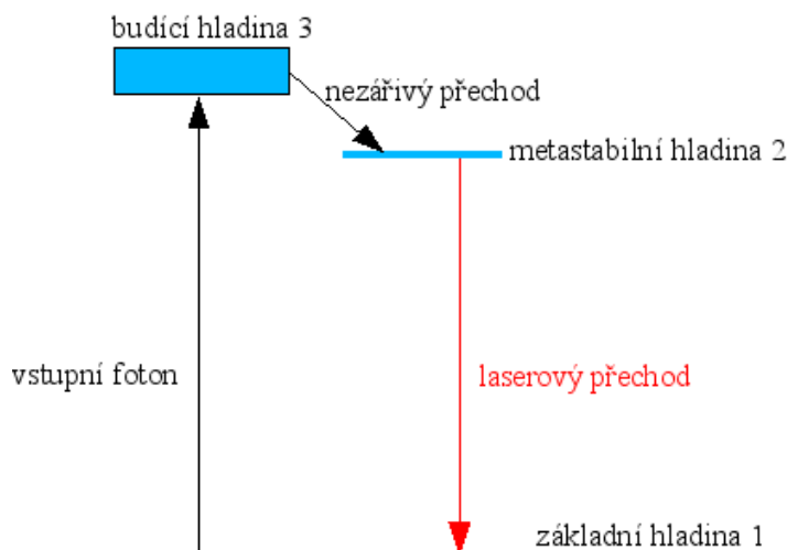
Obr. 3 Metastabilní hladina [9]
