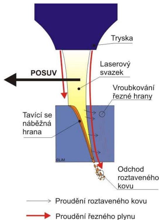
Obr. 13 Řezný proces [8]
