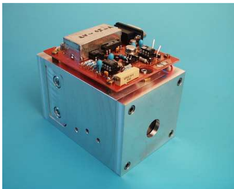
Obr. 12 Polovodičový laser [13]
