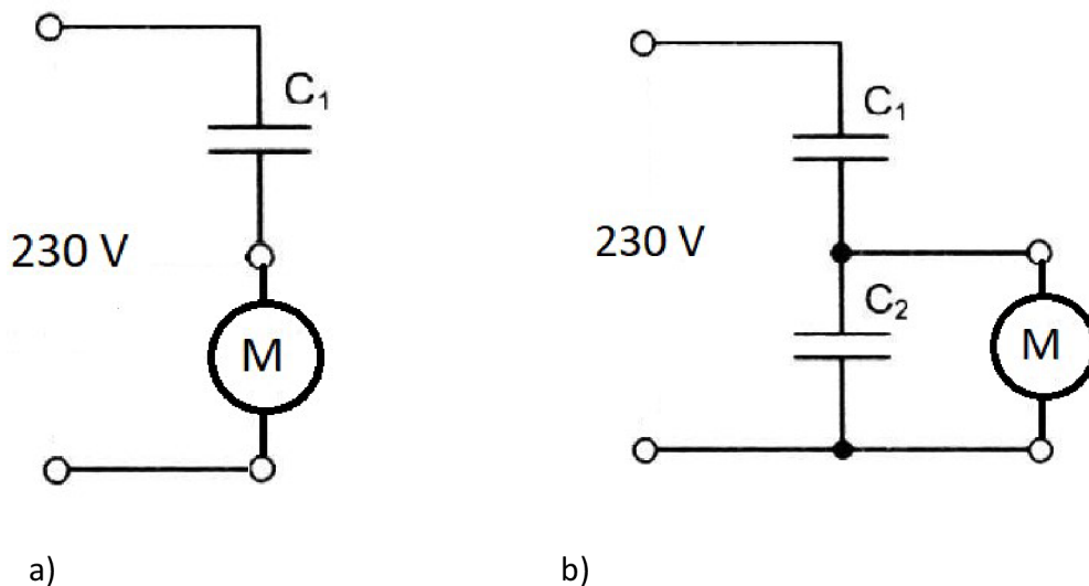
obr. č. 42 Zapojení motorku s kondenzátory. a) Sériové zapojení motorku s kondenzátorem. b) Kapacitní napěťový dělič s připojeným motorkem. Motorek M, kondenzátor C1 a C2. Archiv autora.
