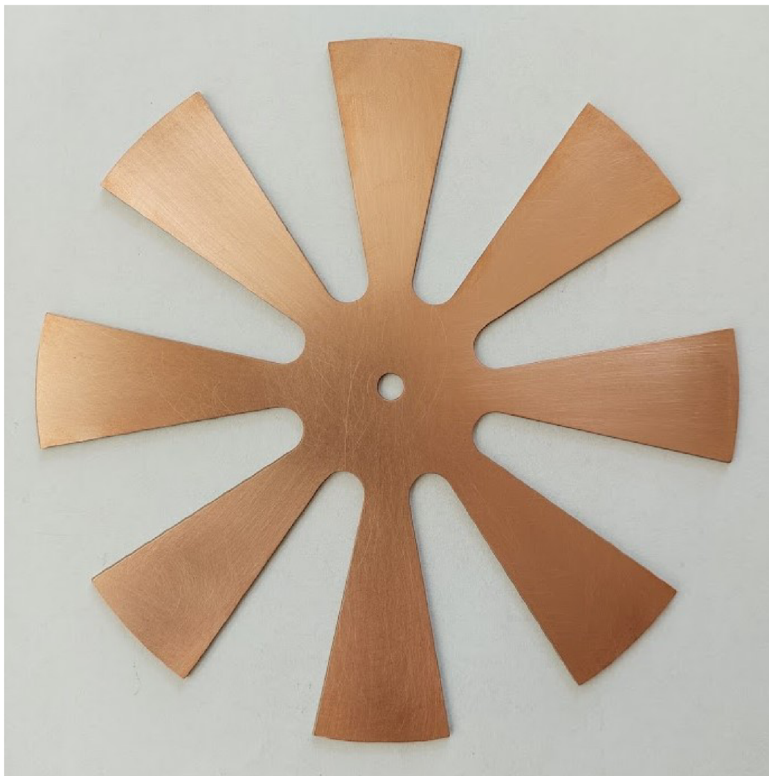
obr. č. 6 Osmilistá rotační stínící elektroda navržena a vyrobena v rámci této práce. Archív autora.
