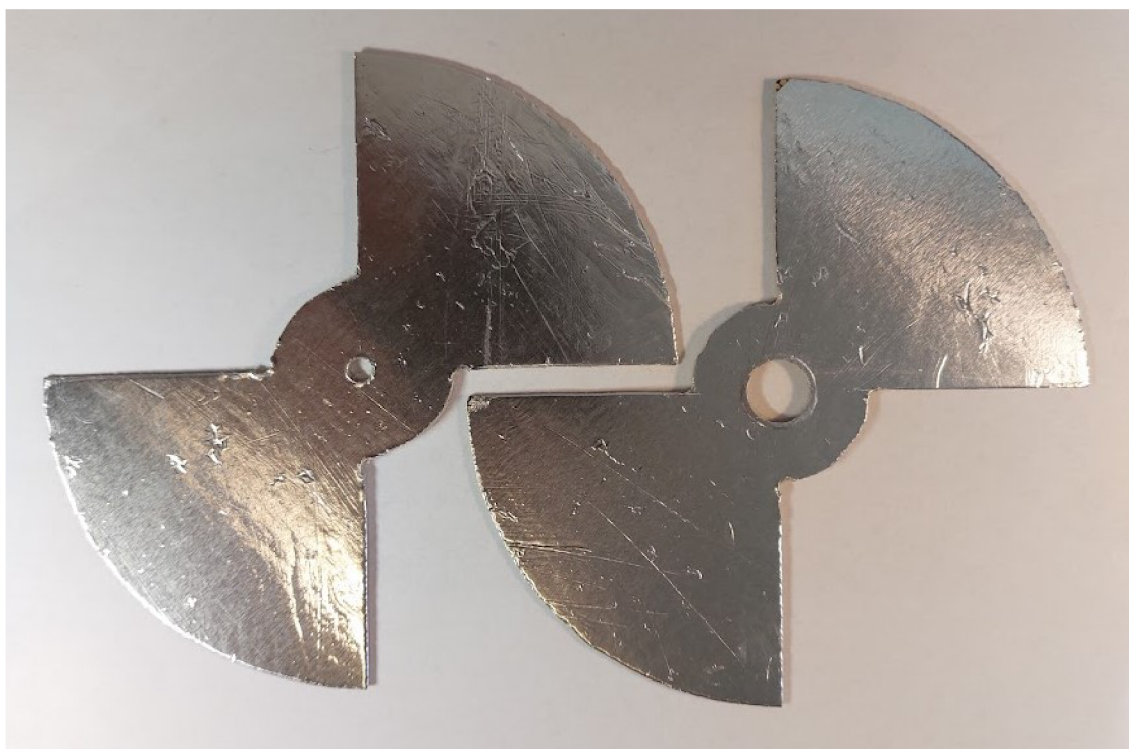
obr. č. 12 Dvoulistá elektroda. Na obrázku vlevo rotační stínící elektroda, na obrázku vpravo stacionární měřicí elektroda. Archív autora.
