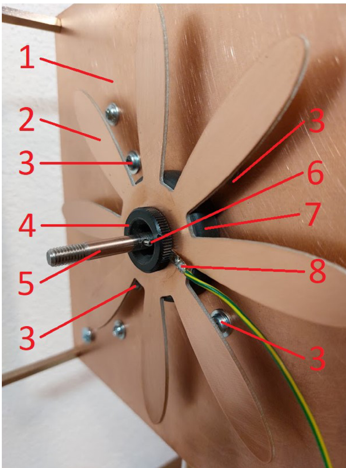
obr. č. 33 Pohled na namontovanou měřící elektrodu na základnu stíněné klece. základna stíněné klece č. 1, měřící elektroda č. 2, šroubek M4 (zašroubován do mezikusu za základnou) č. 3, dutý plastový šroub č. 4, hřídel motorku č. 5, příčný kolík hřídele motorku č. 6, distanční podložka měřící elektrody č. 7, očko s otvorem o průměru 16 mm s připojeným vodičem č. 8. Archív autora.
