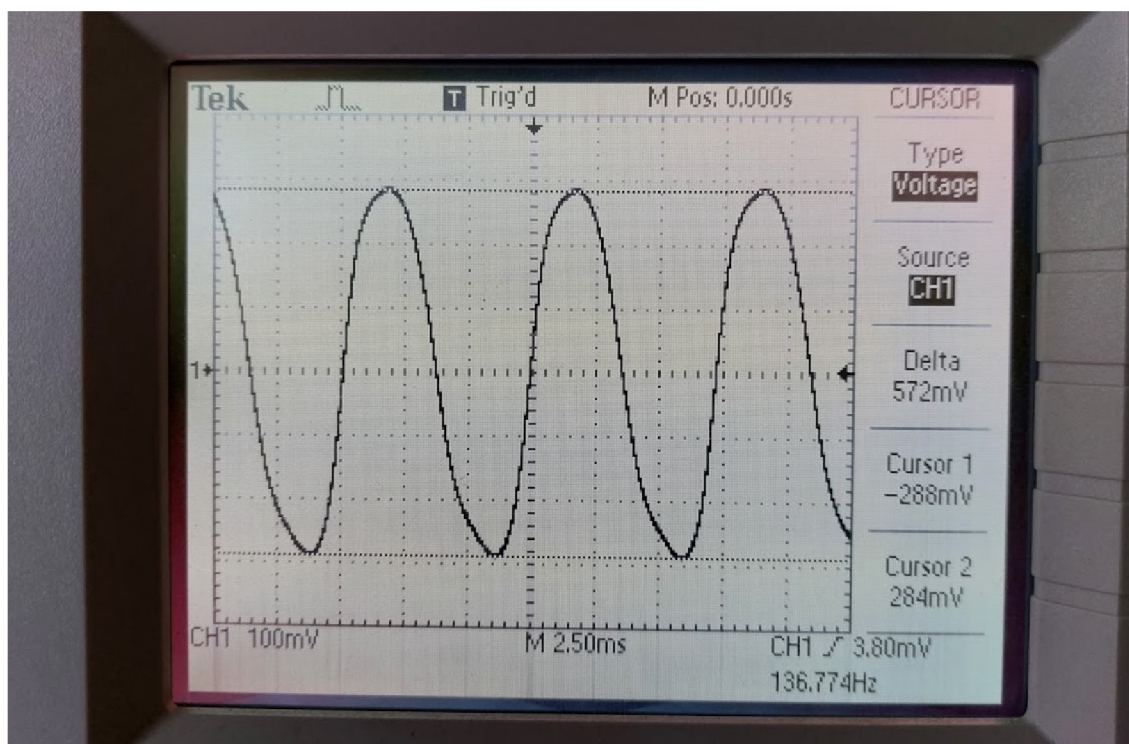
obr. č. 55 Generované napětí třílistou měřicí elektrodou při napětí 7,5 kV. Archív autora.
