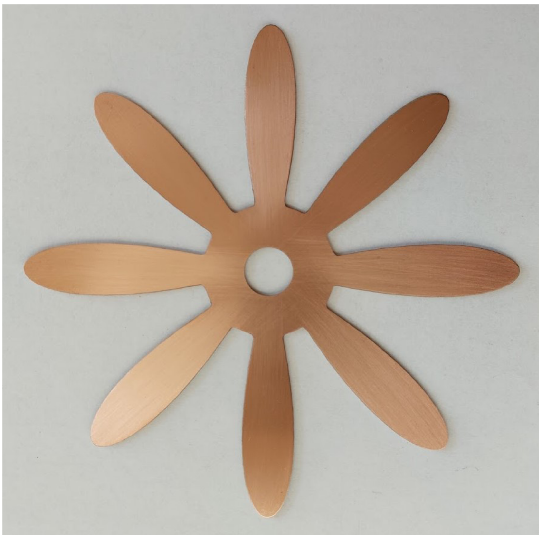
obr. č. 5 Osmilistá stacionární měřicí elektroda navržená a vyrobená v rámci této práce. Archív autora.
