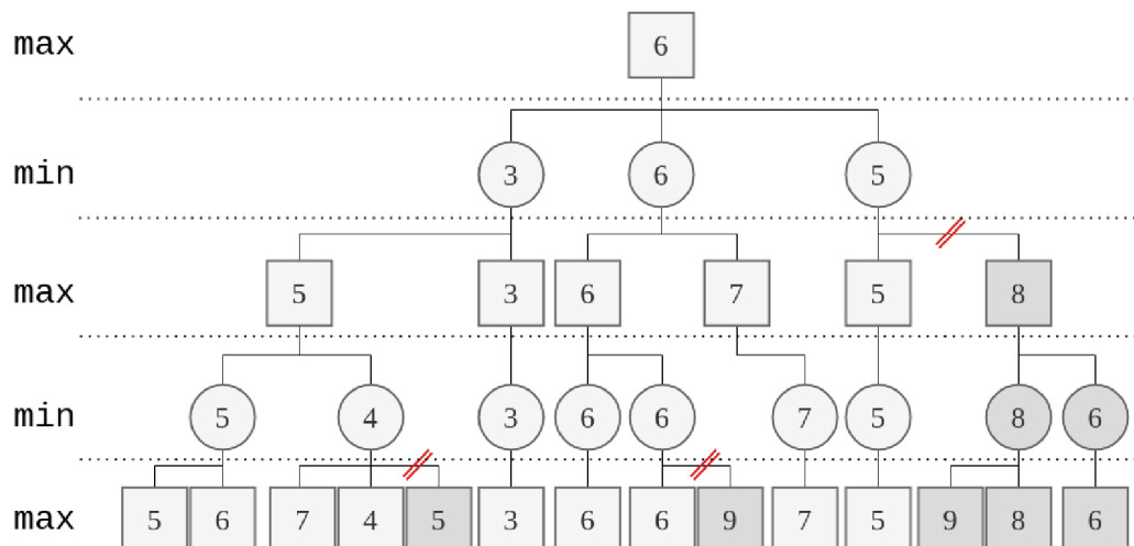
Obrázek 3.2: příklad Alfa-beta ořezávání, ořezané uzly jsou v šedé
