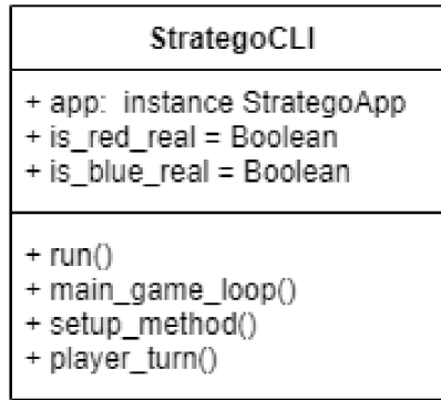
Obrázek 6.1: Třídní diagram StartegoCLI
