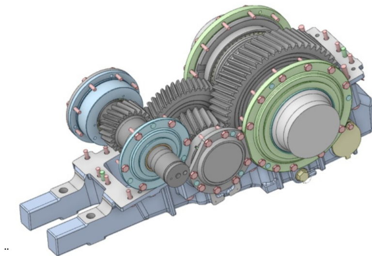
Obrázek 2.7: Model čelní dvoustupňové nápravové převodovky bez horní části skříně
