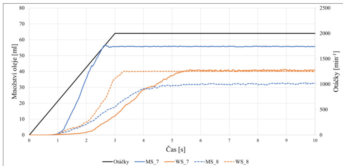
Obrázek 10.29: Změna množství oleje ve sběrných kapsách v průběhu simulace sedmého a osmého výpočetního modelu
