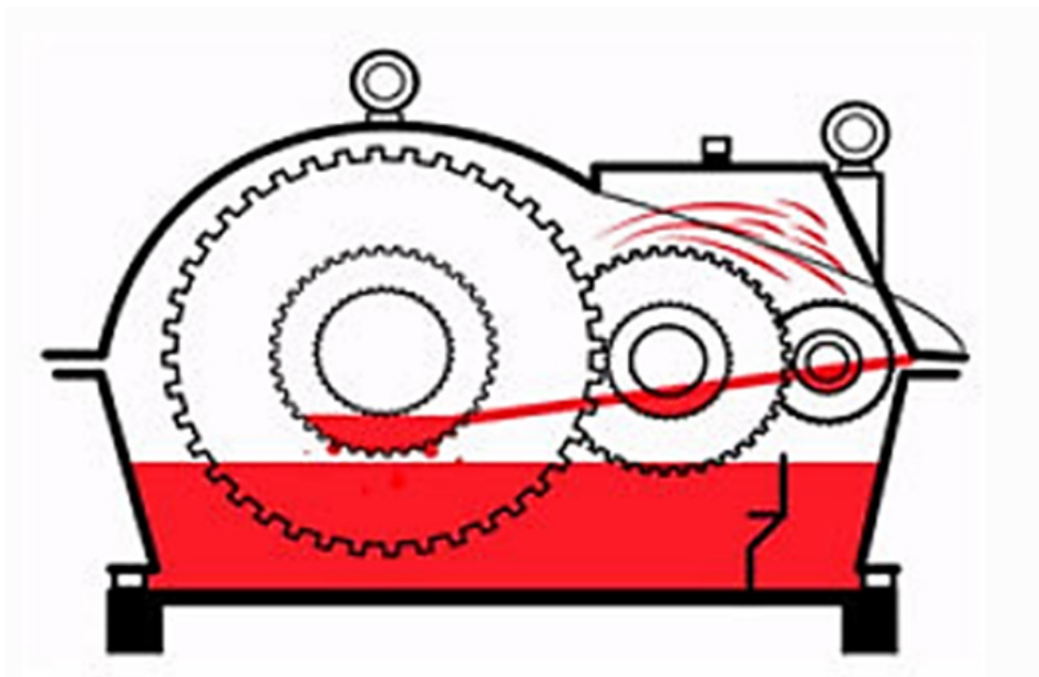
Obrázek 3.2: Mechanismus mazání rozstříkem[18]
