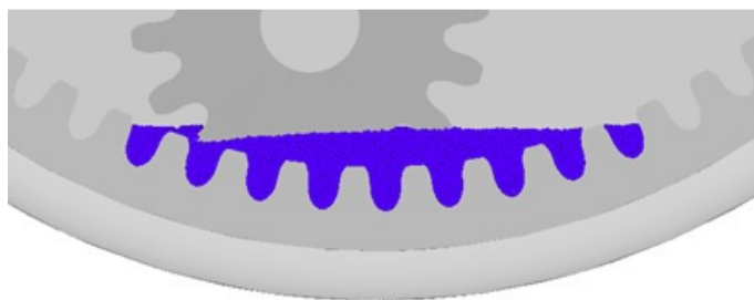
Obrázek 8.2: Výška hladiny při ponorné hloubce kola 3\cdot m_n
