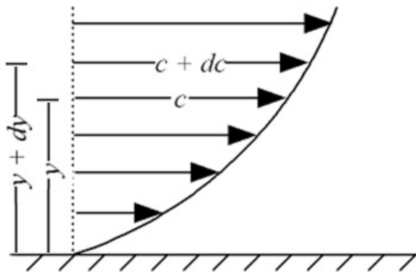
Obrázek 3.5: Smykového napětí při pohybu kapaliny [25]
