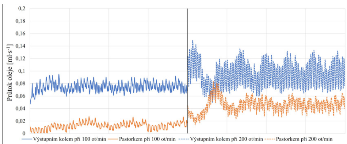
Obrázek 9.2: Průtok oleje vnesený koly při ponorné výšce 3 \cdot m_n po dobu 2 s. Vlevo při 100 \text{ min}^{-1} a vpravo při 200 \text{ min}^{-1}
