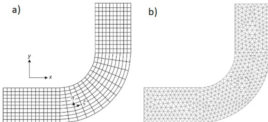
Obrázek 5.6: Strukturovaná síť a), Nestruturovaná síť b) [31]
