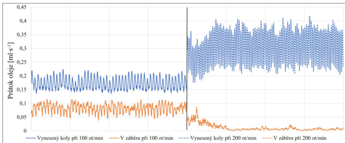
Obrázek 9.6: Porovnání průtoku oleje záběrem vůči celkovému vyneseny koly při ponorné výšce 6 \cdot m_n po dobu 2 s. Vlevo při 100 \text{ min}^{-1} a vpravo při 200 \text{ min}^{-1}
