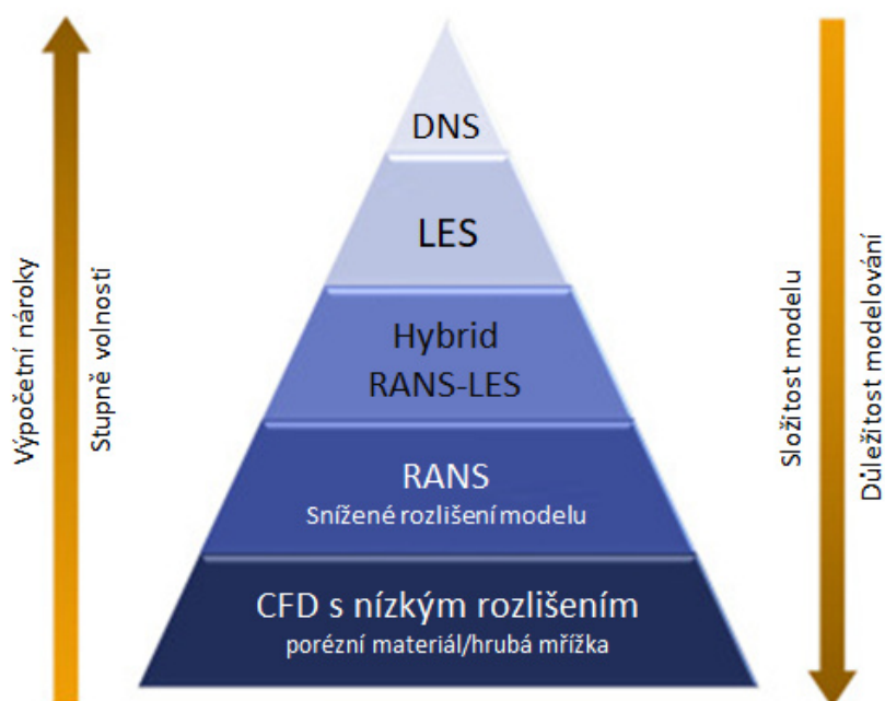
Obrázek 5.1: Modely turbulence [34]
