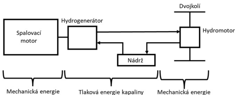
Obrázek 2.3: Hydrostatický přenos výkonu [6]
