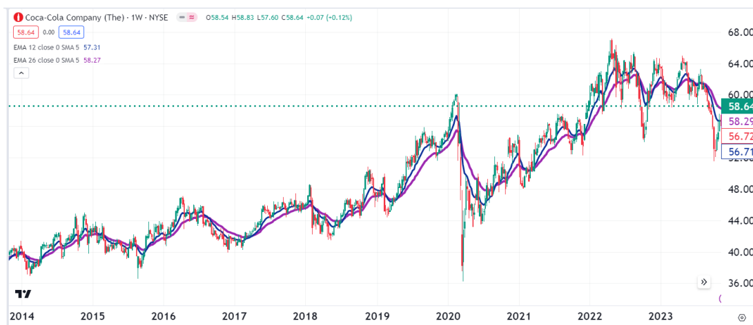
Obrázek 1 Krátkodobý a dlouhodobý exponenciální klouzavý průměr aplikovaný pro akcie firmy Coca-Cola Company v období 10 let
