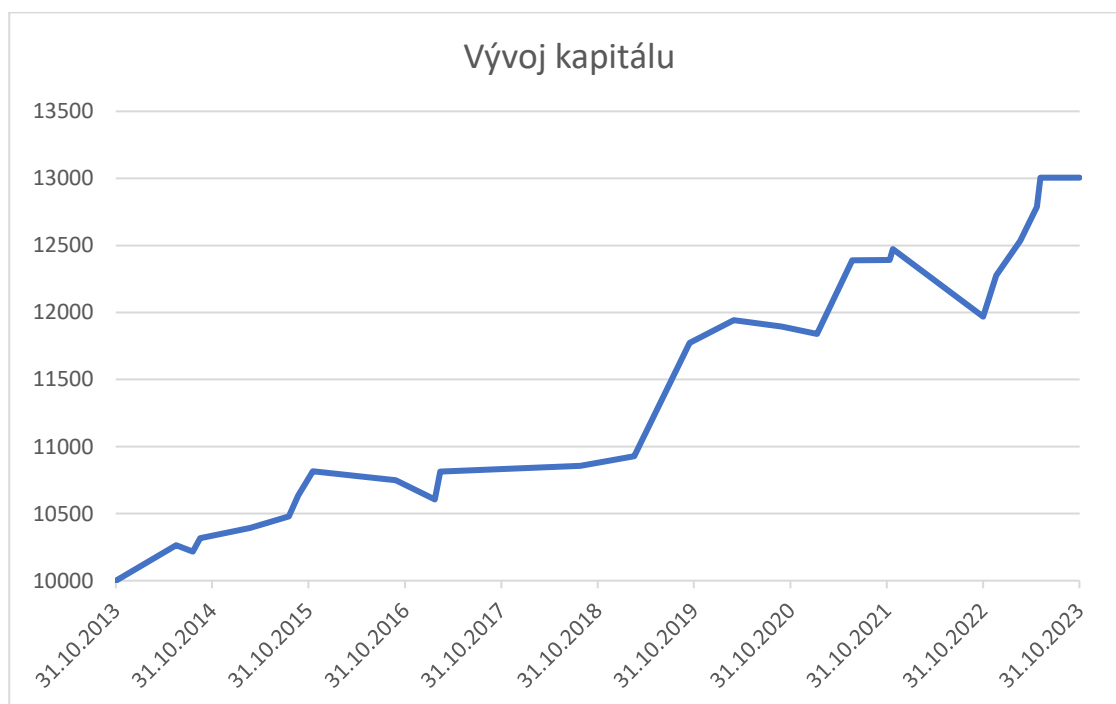
Graf 1 Strategie RSI vývoj obchodního kapitálu
