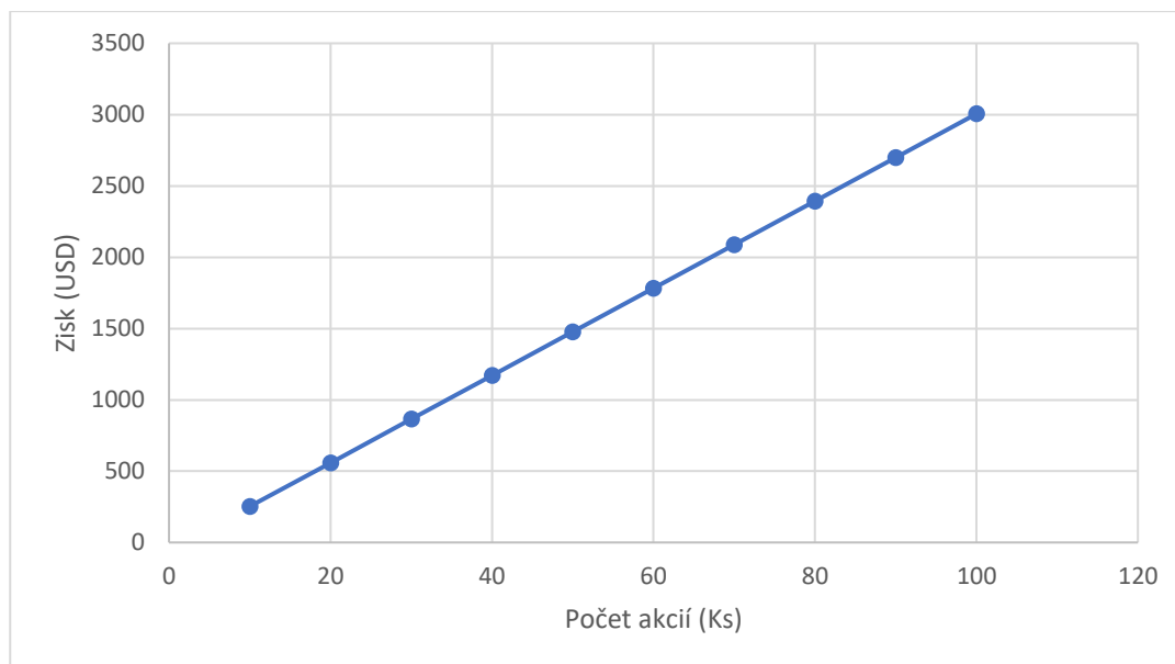
Obrázek 8 Vývoj zisku při nákupu většího počtu akcií na kontrakt se započítanými dividendami a brokerskými poplatky u modifikované strategie RSI
