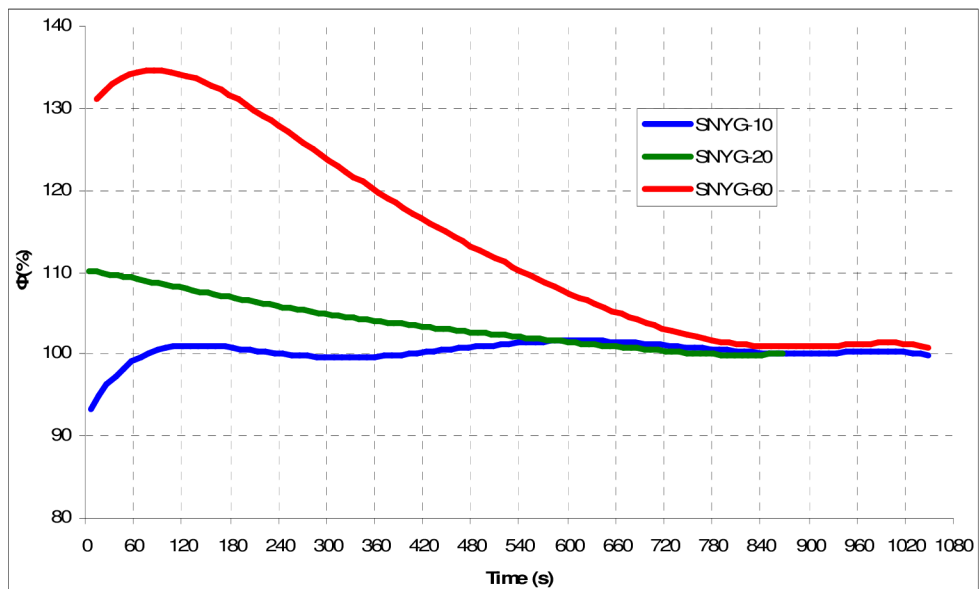
Obr. 4-3 Náběh světelného toku bezelektrodevých zářivek série SNYG [9]
