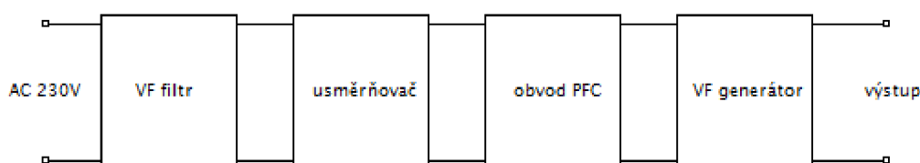
Obr. 4-1 Blokové schéma předřadného systému pro bezelektrodové zářivky
