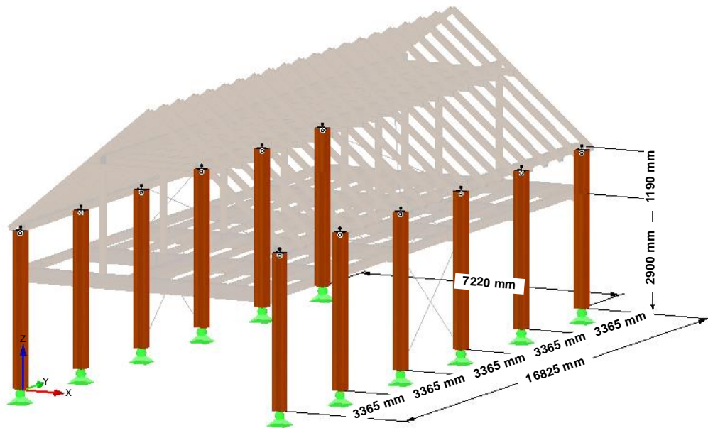
Obrázek 7 - Sloupy 240x320 mm
