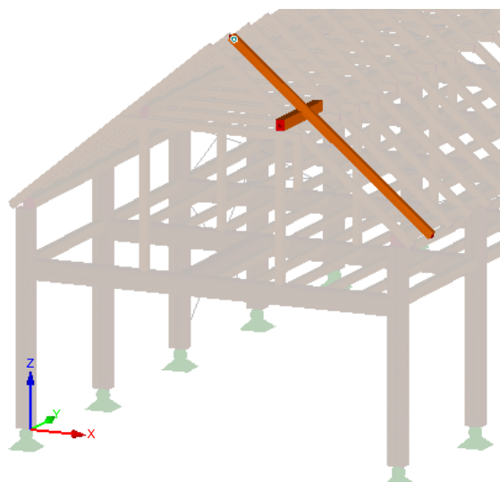
Obrázek 29 - DETAIL 2
