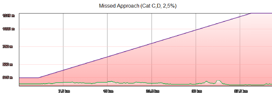
Obr. M – výškový profil postupu dle GE (složení a úprava 2 zobrazení)
