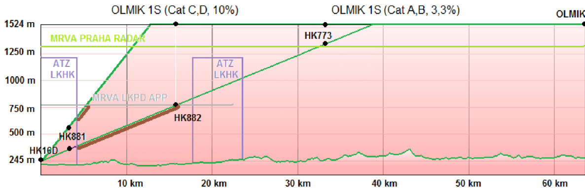
Obr. 23 – výškový profil postupu dle GE (složení a úprava 2 zobrazení)
