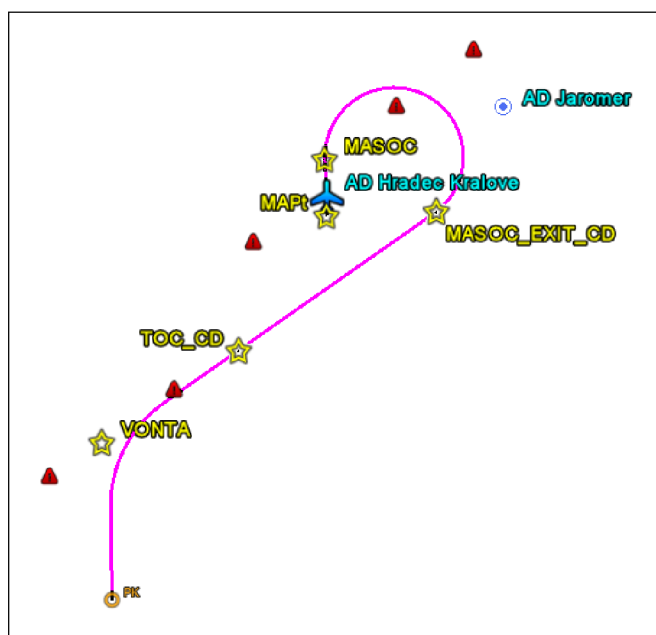
Obr. 14 – náčrt postupu nezdařeného přiblížení
