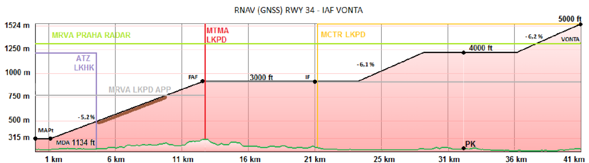
Obr. 20 – výškový profil postupu dle GE (složení a úprava 2 zobrazení)
