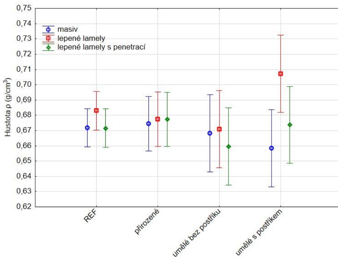
Graf 7. Změna hustoty v závislosti na způsobu stárnutí (autor).
