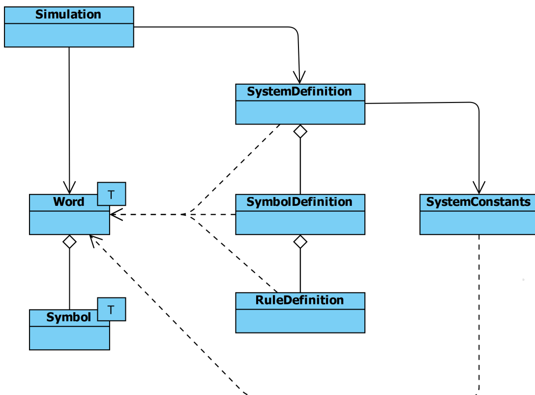
Obrázek 5: Diagram tříd pro práci s L-systemy.
