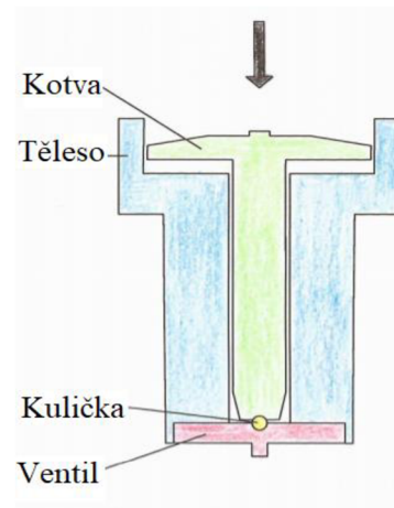
Obr. 25 Interní lisování
