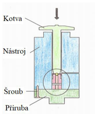
Obr. 23 Externí lisování
