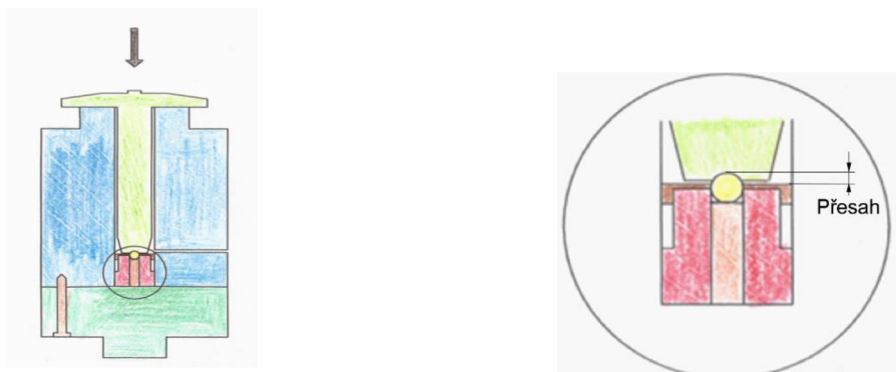
Obr. 26 Nový nástroj pro externí lisování Obr. 27 Detail nového nástroje pro externí lisování
