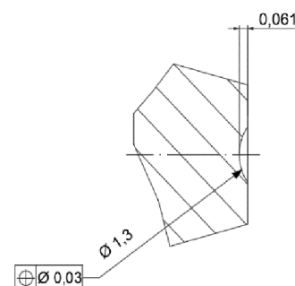
Obr. 22 Otlak kotvy
