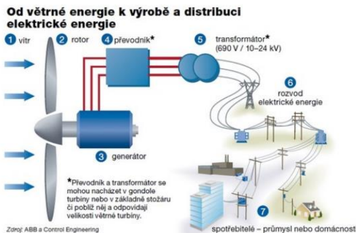
Obr. 22 Schéma výroby a distribuce elektrické energie
