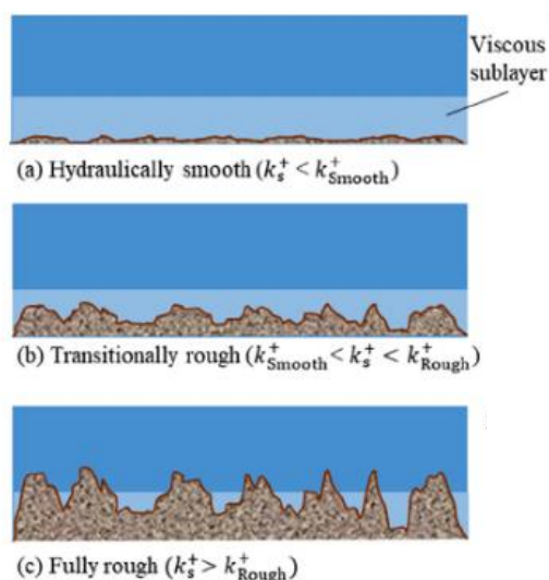
Obr. 10 Turbulentní proudění nad drsné povrchy; (a) hydraulicky hladký režim s drsností uloženu pod viskózní podvrstvou, (b) přechodně drsný režim s částečně rozloženou viskózní podvrstvou, (c) plně drsný povrch s úplně destruovanou viskózní podvrstvou [54]
