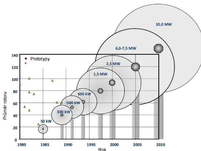
Obr. 14 Průměr rotoru a výkon vrtule [48]
