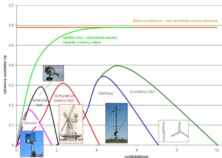
Obr. 24 Výkonový součinitel větrné turbíny, zdroj: ČSVE
