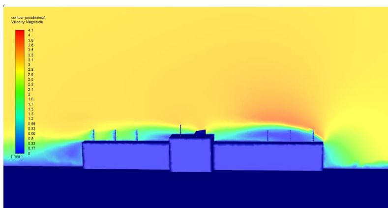
Obr. 55 Obrázek rychlosti proudění větru se střechou a stožáry o výšce 4200 mm
