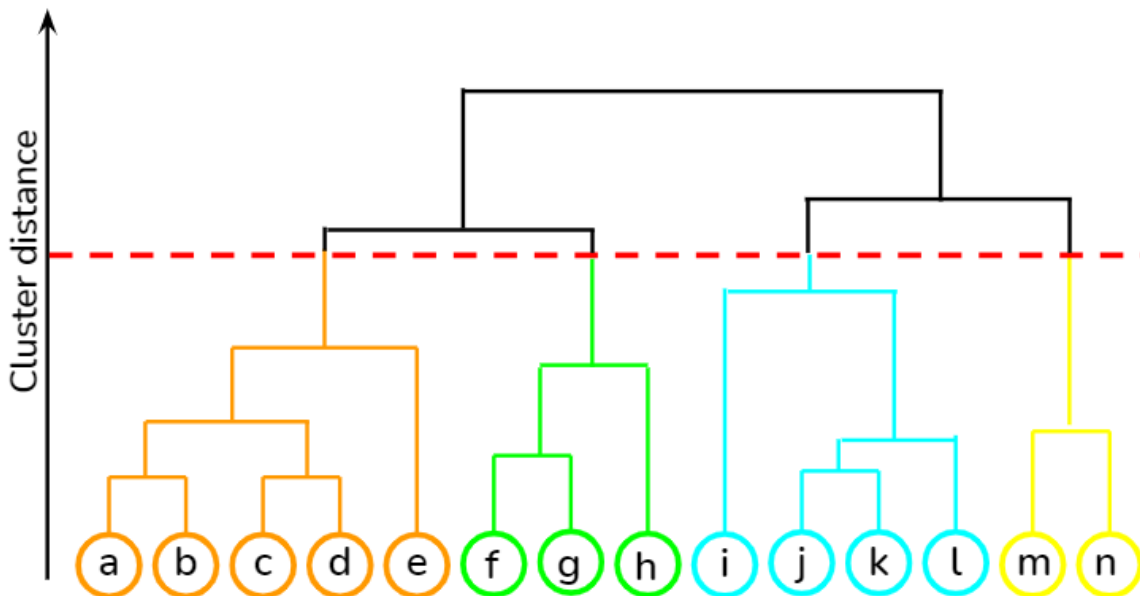
Obrázek 9 - hierarchický clustering
