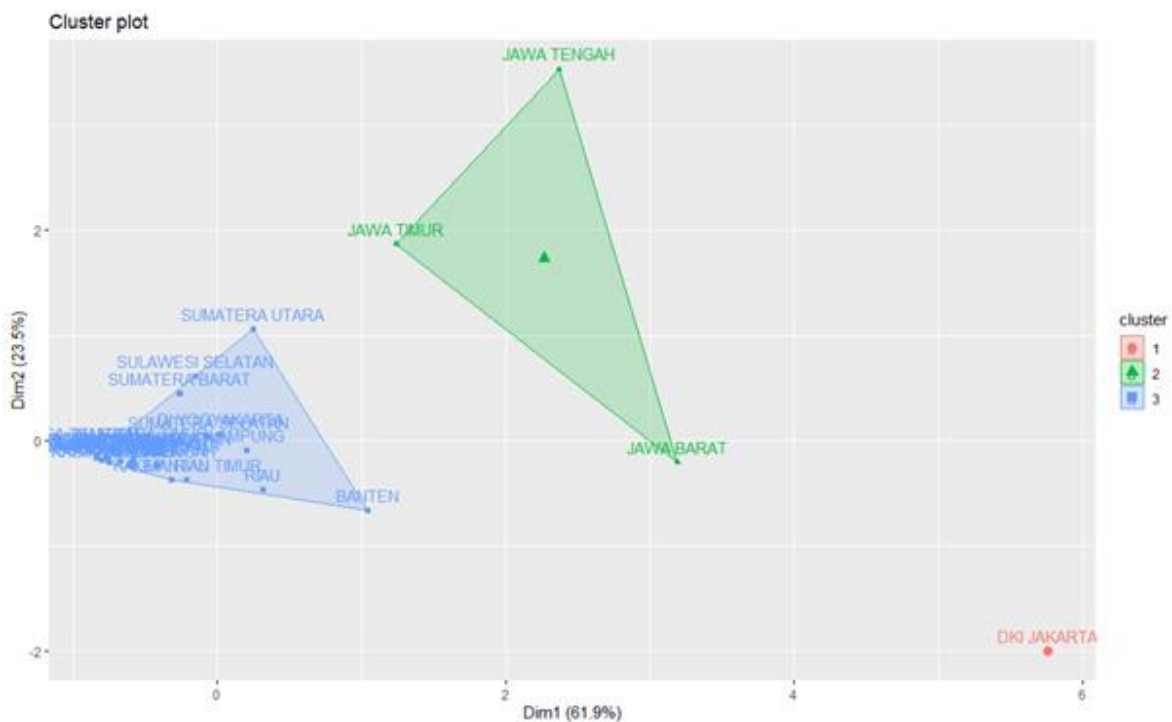
Obrázek 10 - nehierarchický clustering
