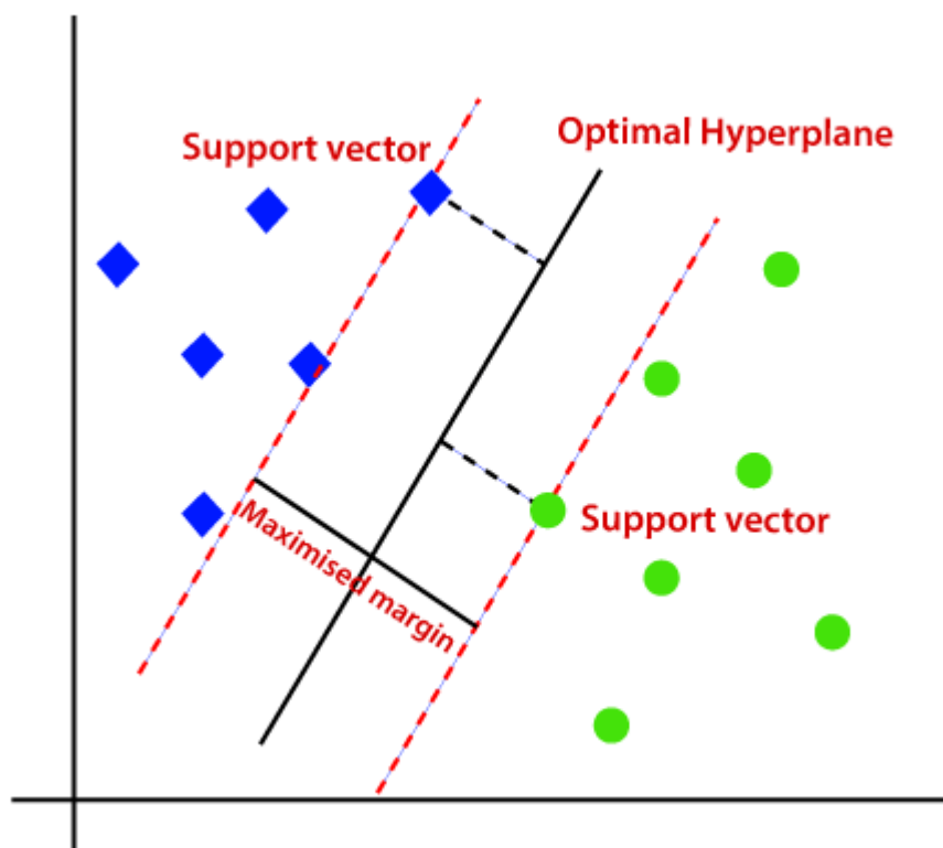
Obrázek 16 - SVM algoritmus
