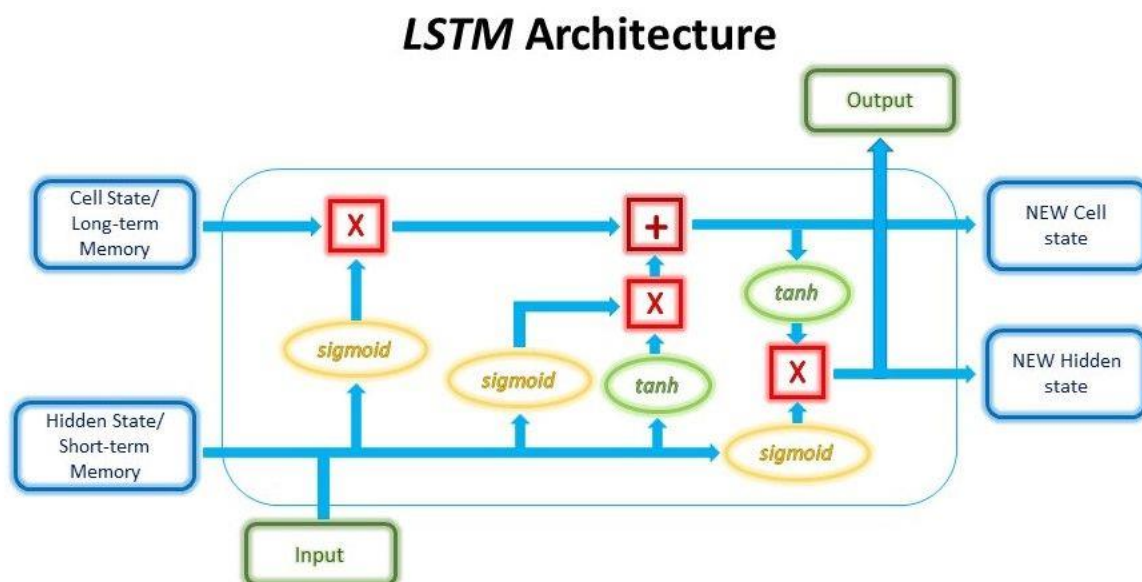
Obrázek 13 - architektura LSTM
