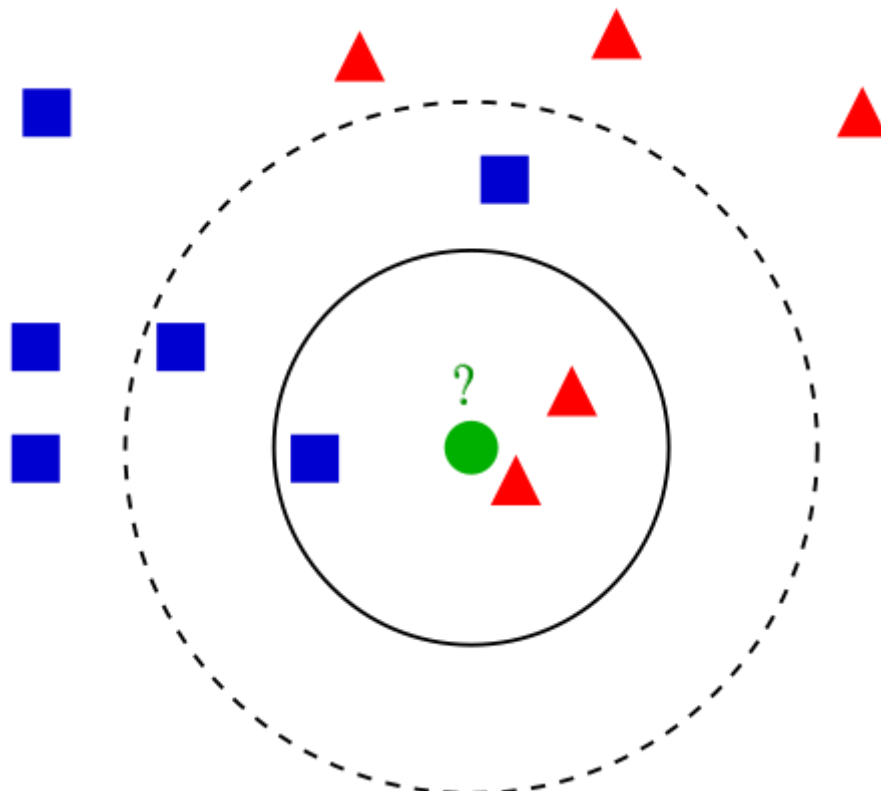
Obrázek 15 - K-NN algoritmus
