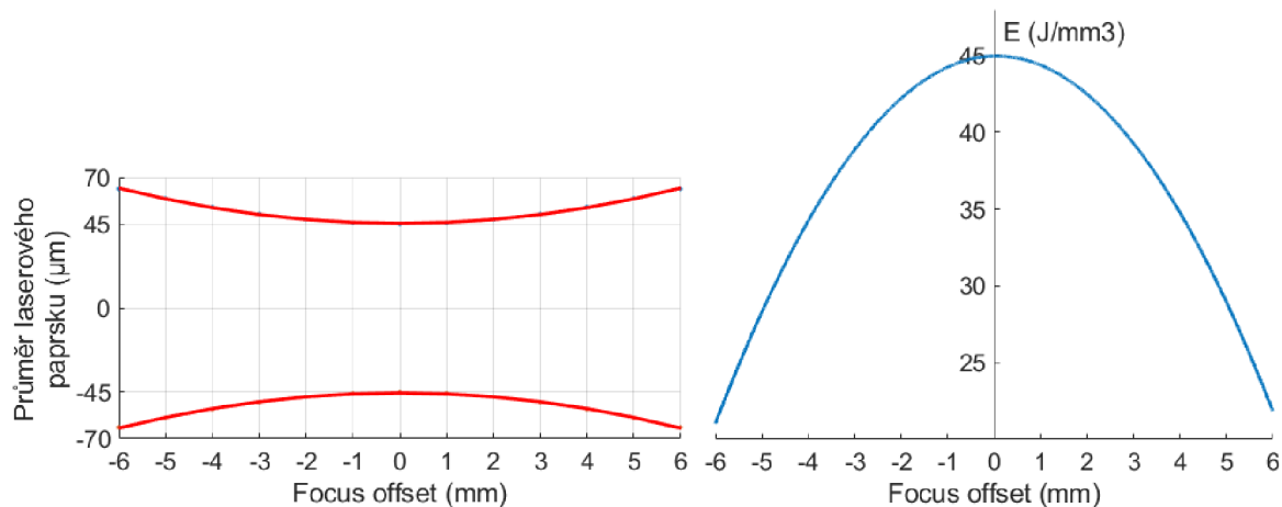
Obr. 5-25 Závislost průměru laserového paprsku (vlevo), a hustoty energie (vpravo) na parametru zaostření
