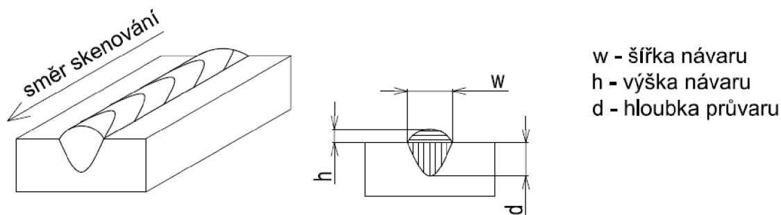
Obr. 4-6 Geometrie návaru
