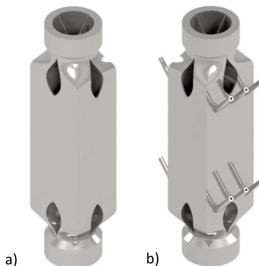
Obr. 4-14 a) Jednoduchá varianta navrženého výměníku; b) varianta s pruty pro odběr statického tlaku
