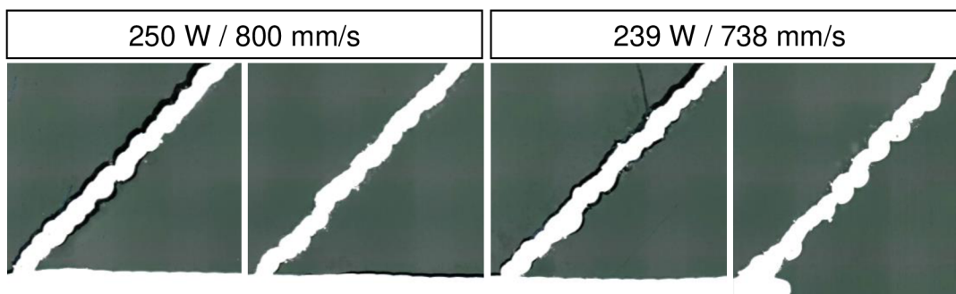
Obr. 5-32 Metalografický výbrus stěny pod úhlem 45° tvořené jedním návarem
