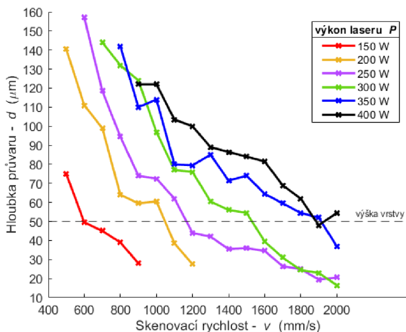
Obr. 5-8 Závíslost hloubky průvaru na rychlosti skenování
