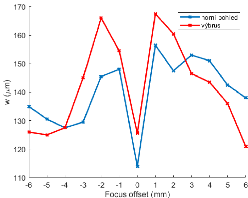
Obr. 5-30 Šířka návaru se změnou zaostření
