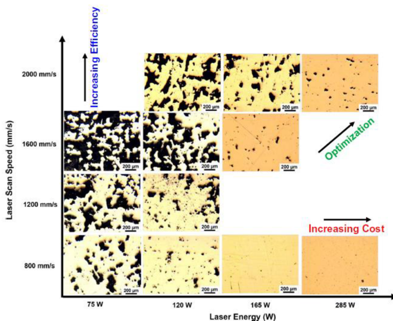
Obr. 2-15 Optické mikrografy porozity vzorků jako funkce výkonu a rychlosti [28]
