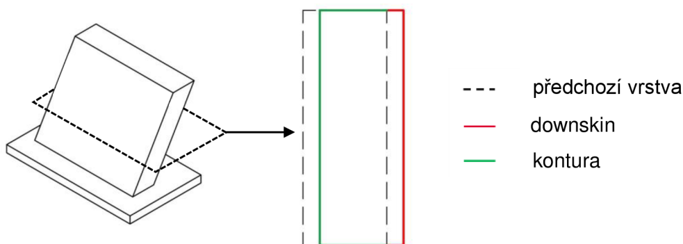
Obr. 4-10 Rozdělení skenovací oblasti parametrem downskin v rámci jedné vrstvy
