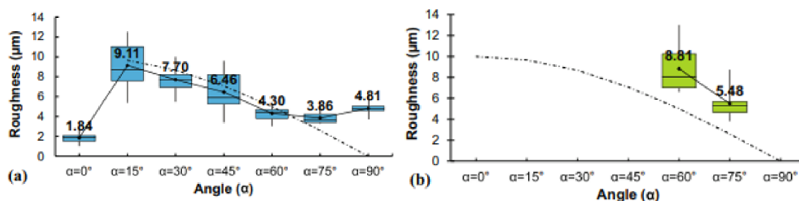
Obr. 2-10 Závislost drsnosti povrchu na úhlu; a) horní povrch; b) spodní povrch; [25]
