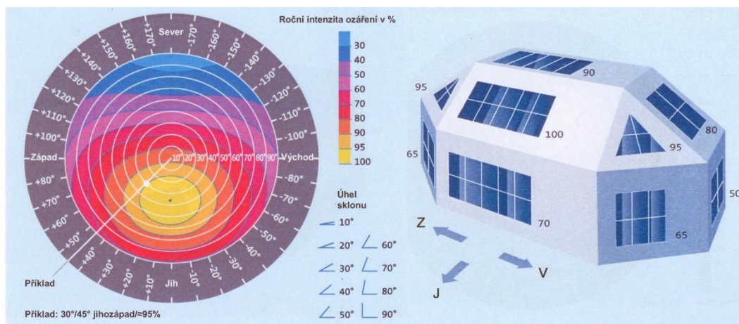
Obrázek 15: Pomůcka pro rychlou orientaci výkonu FVE (aeko s. r. o. 2022).
