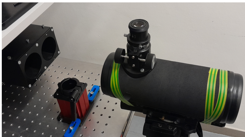
Obrázek 3.1: Měřící teleskop pro ověření souososti.
