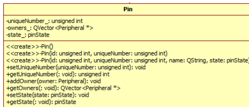
Obrázek 4.7: Náhled na třídu Pin.
