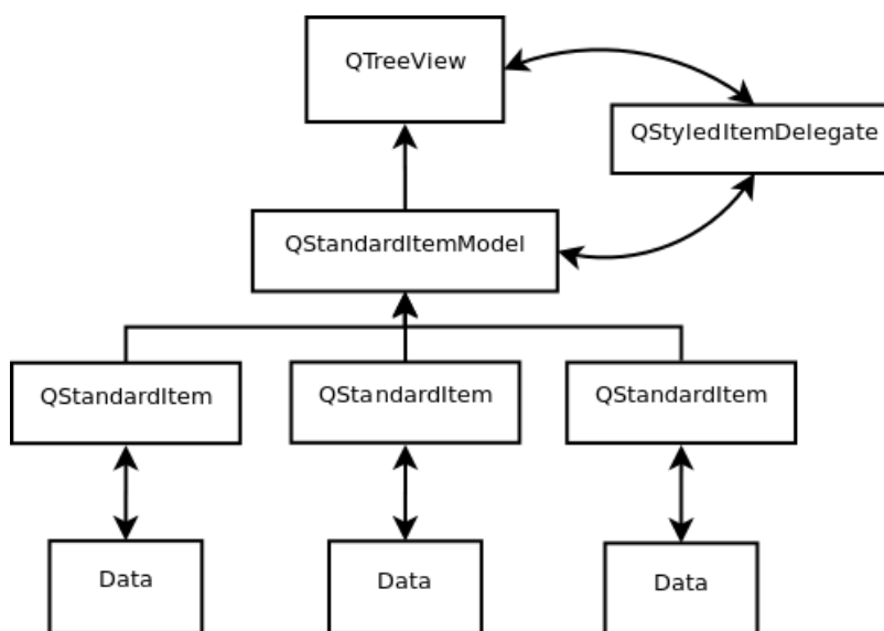
Obrázek 5.2: Pozice delegáta Při model-view programování v Qt.
