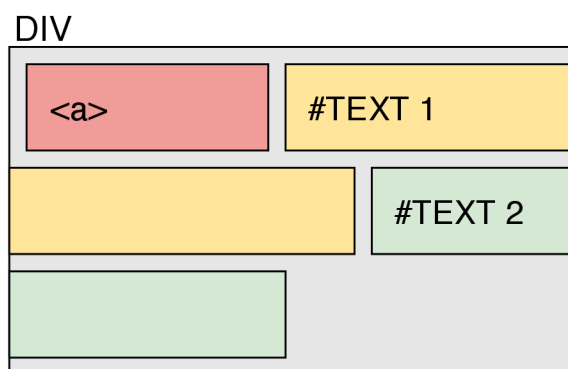
Obrázek 5.4: I když to na obrázku není zobrazeno, tak odkaz obsahuje taky textový element. Nejprve se zpracuje <a> . Poté se začne Text1, který pozici nebude zjišťovat z nadřazeného uzlu jak u minulého příkladu, ale zjistí pozici a rozměr posledního přidaného textového elementu. Posledním přidaný text je z odkazu. Vypočítá se nová pozice pro Text1. Text2 se připojí k Textu1 jako v minulém příkladu.
