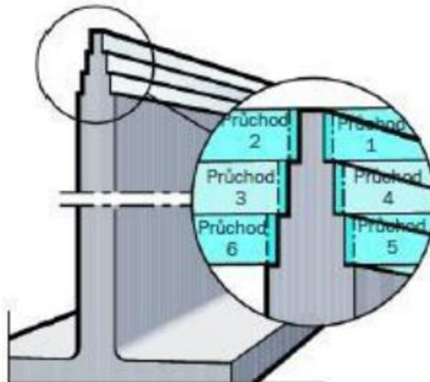
Obr. 40 Postup při frézování velmi tenkých stěn [38].
