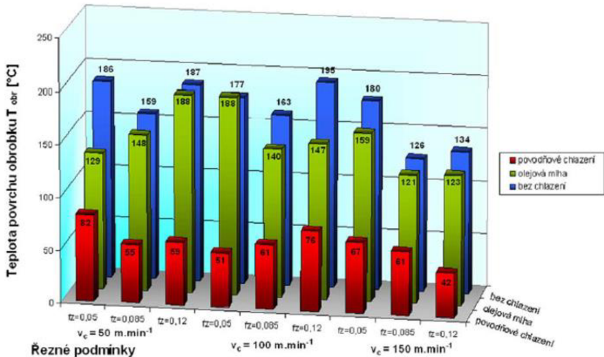
Obr. 29 Závislost teploty obrobené plochy na rezných podmínkách při frézování slitiny Ti6Al4V [32].
