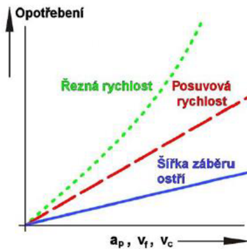
Obr. 7 Vliv řezných podmínek na opotřebení [1].
