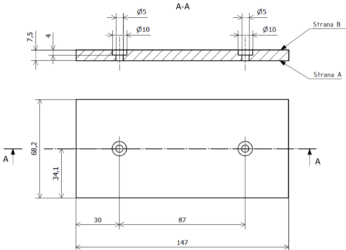
Obr. 47 Rozměry vzorků.
