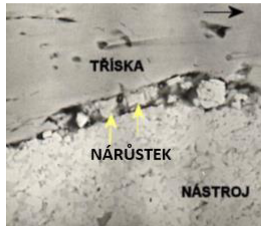
Obr. 5 Nárůstek a působení třísky [1].
