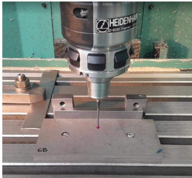
Obr. 49 Měření rovinnosti vzorku pomocí dotykové sondy v upnutém stavu.
