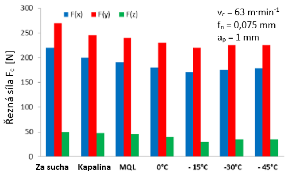
Obr. 31 Vliv řezného prostředí na silové zatížení nástroje [34].
