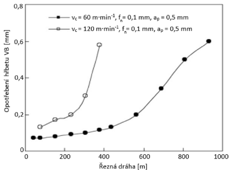
Obr. 24 Grafická závislost opotřebení na řezné dráze [25].
