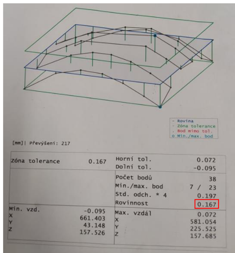
Obr. 46 Protokol z měření rovinnosti po obrobení jedné strany při upnutí lepidlem.
