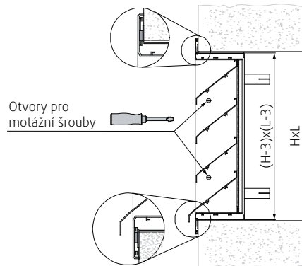
Obr. 1: Detaily žaluzie
