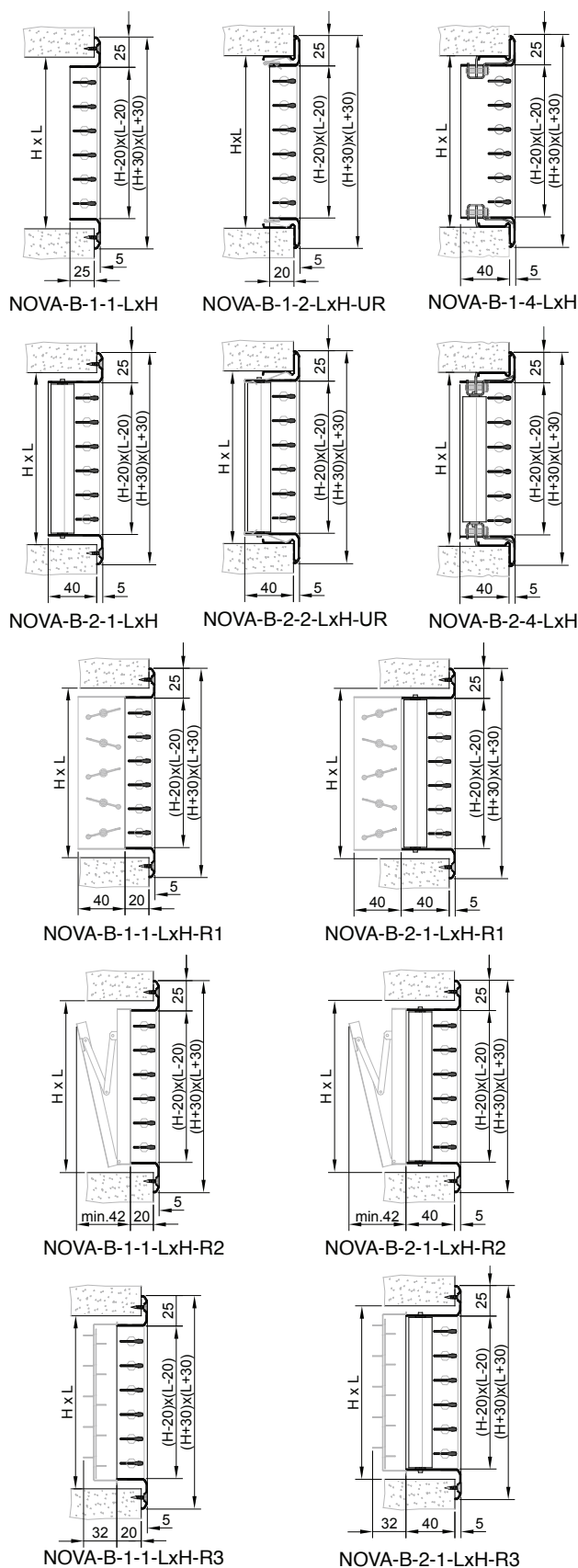
Obr. 1: Rozměry vyústky
