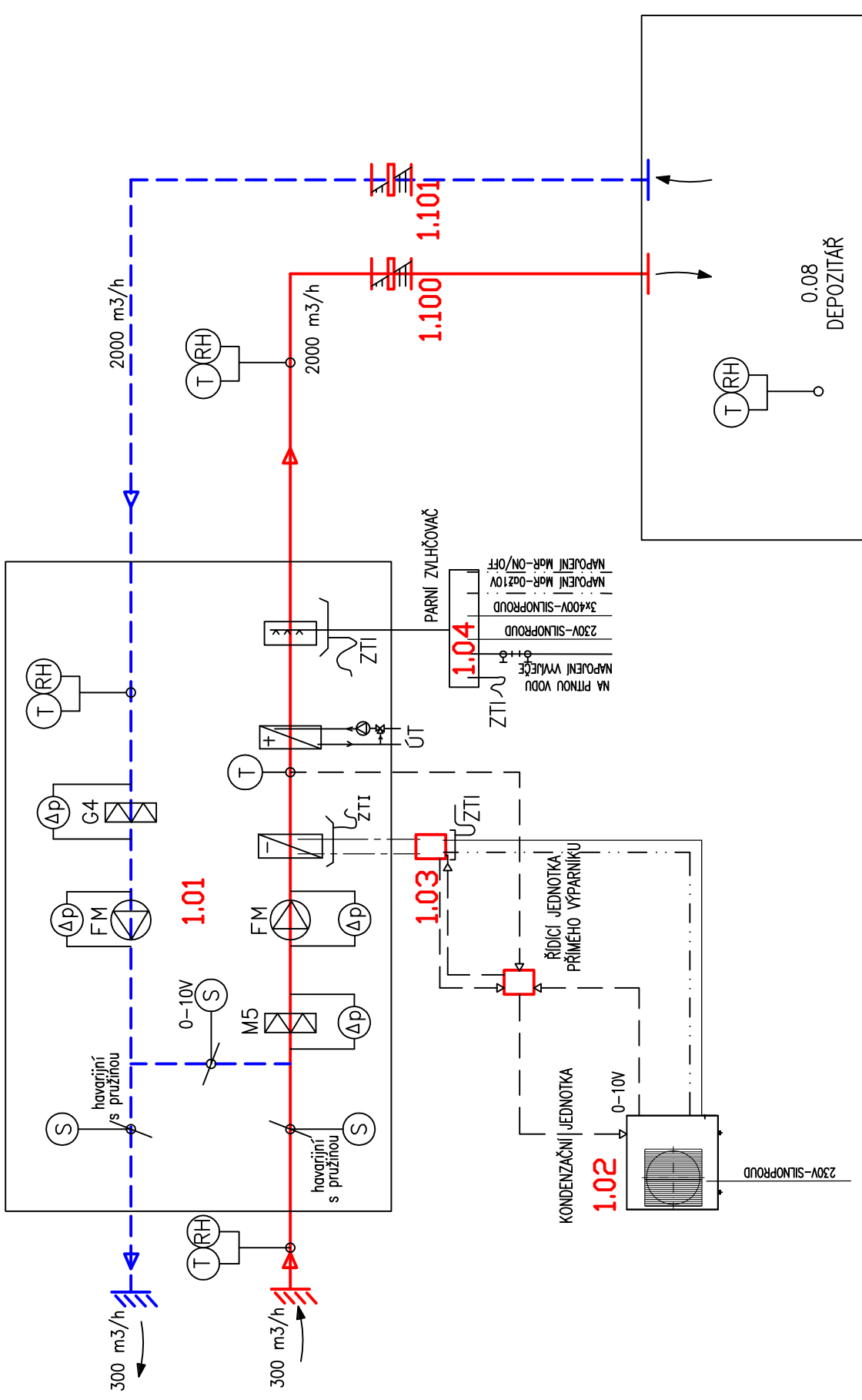
FUNKČNÍ SCHEMA
