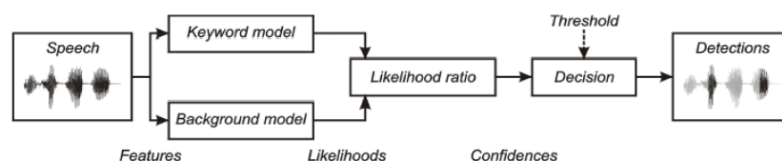
Obrázek 2.2: Schéma procesu rozpoznávání klíčových slov [13]
