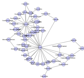
Obrázek 5.1: Vztahová síť 1
