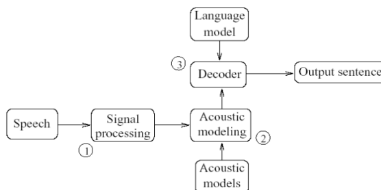
Obrázek 2.3: Schéma procesu přepisu řeči na text [13]
