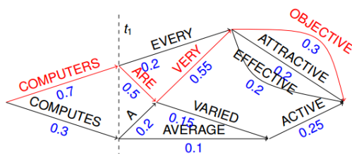
Obrázek 2.4: Příklad výstupního grafu hypotéz (lattice) [6]
