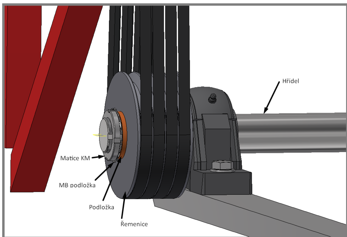
Obr. 44 Způsob upevnění druhé řemenice na hřídeli
