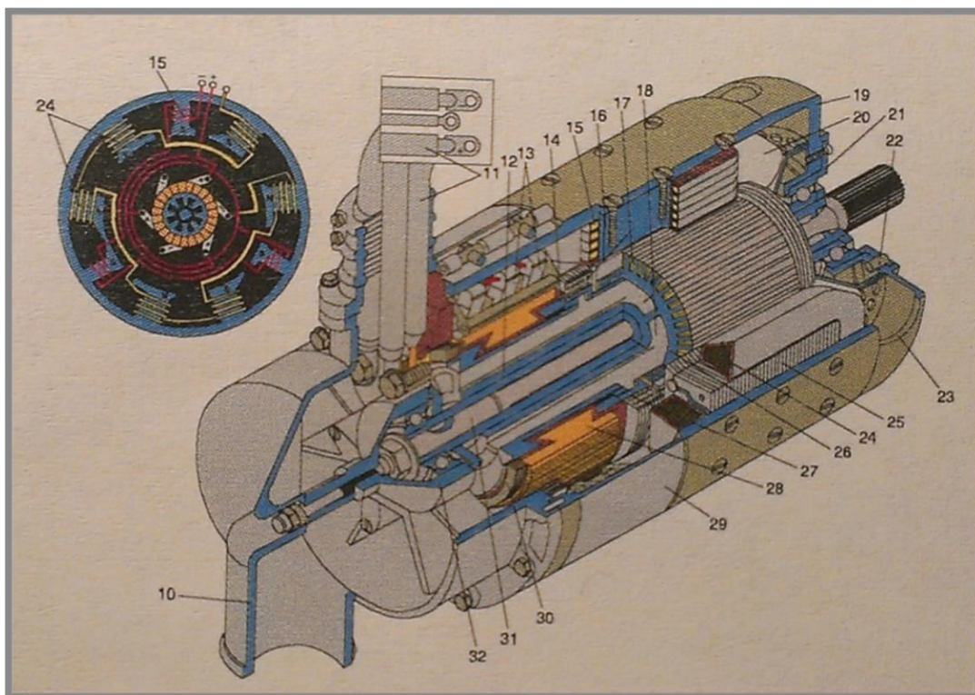
Obr. 8 Schéma dynama G6,5-S
