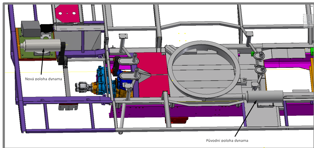
Obr. 25 Umístění dynamo a převodů
