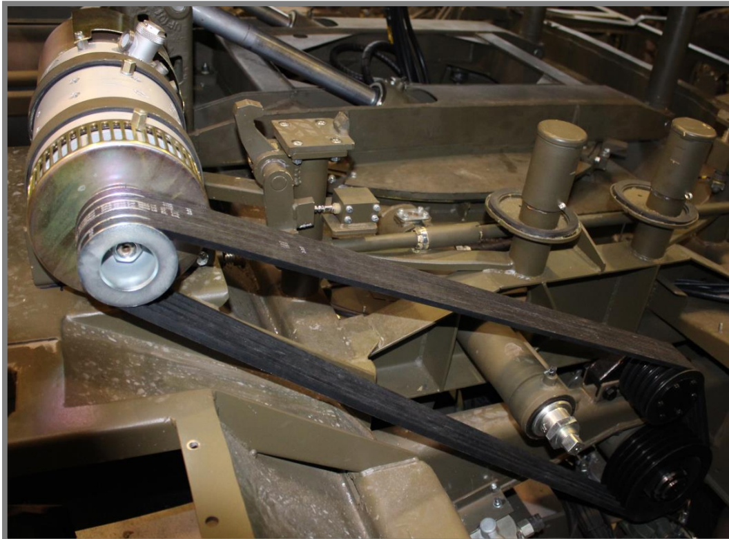
Obr. 18 Současný způsob napínání řemenů
