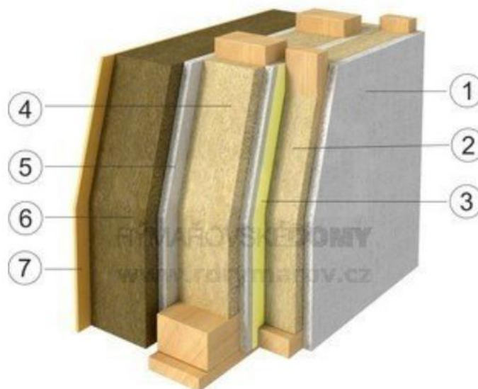
Obrázek 9 – Skladba difúzně otevřené obvodové stěny RD Rýmařov s.r.o. [zdroj: 16]
