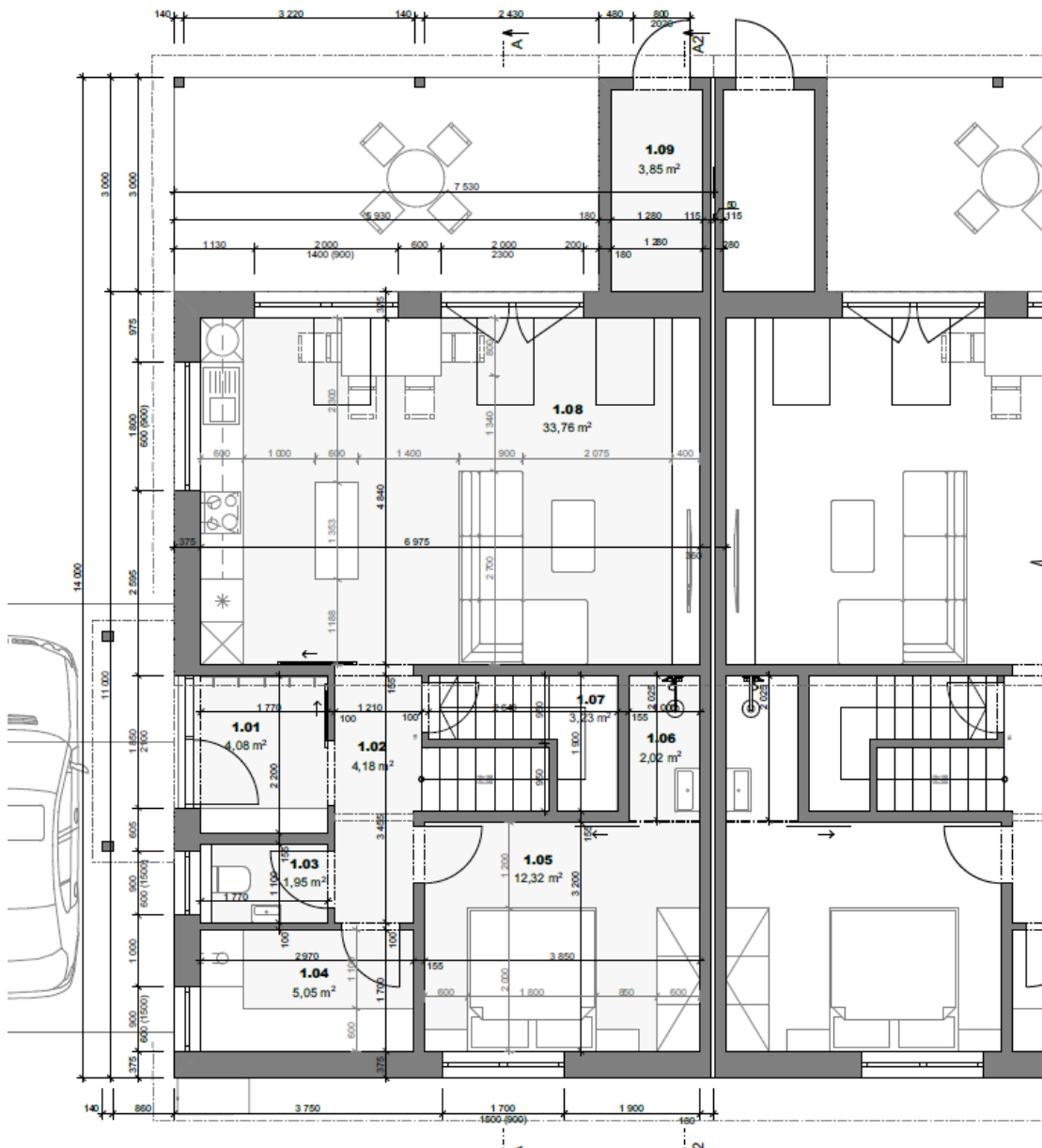
Obrázek 17 - Půdorys 1. NP [autor]
