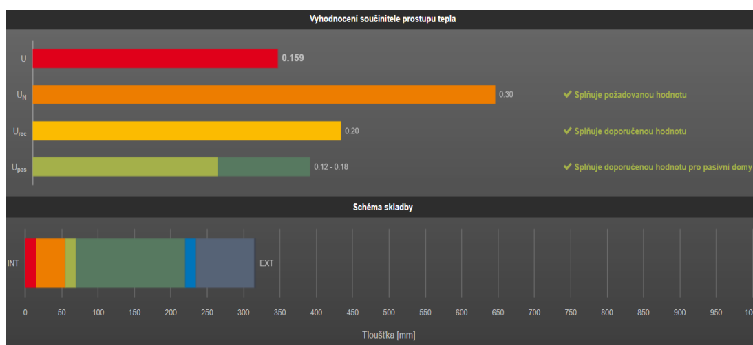
Obrázek 24 – Grafické znázornění výpočtu součinitele prostupu tepla pro STN 7 [autor]
