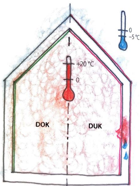
Obrázek 4 - DOK umožňují prostup suchého vzduchu a vodní páry mechanismem difúze, naopak difúzně uzavřené konstrukce (DUK) tento efekt neumožňují. [15, s. 112]
