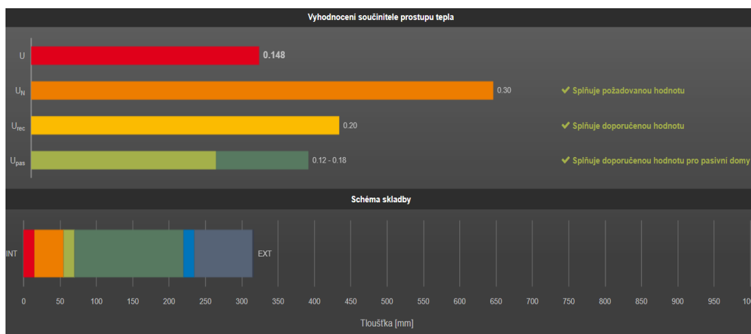
Obrázek 19 – Grafické znázornění výpočtu součinitele prostupu tepla pro STN 2 [autor]
