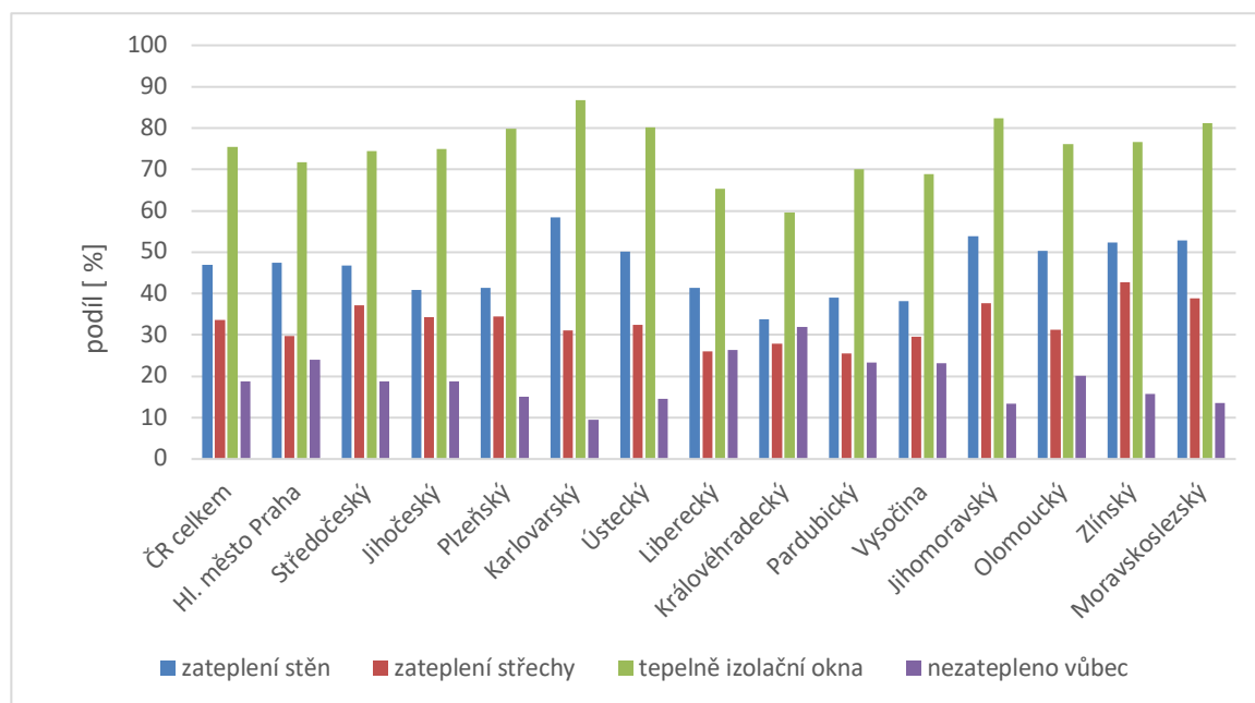
Obrázek 1 - Ukazatel jednotlivých zateplení podle krajů ČR [6]
