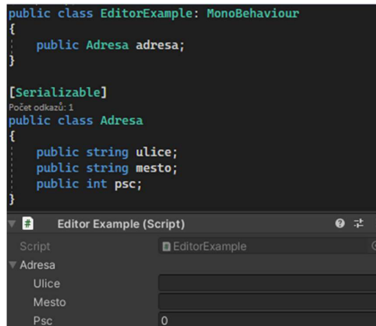
Obrázek 37 - Příklad serializované třídy bez PropertyDrawer
