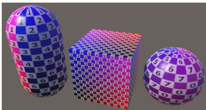
Obrázek 61 - UV Mesh
