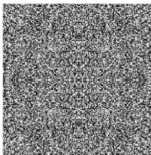
Obrázek 2 - Normal Noise
