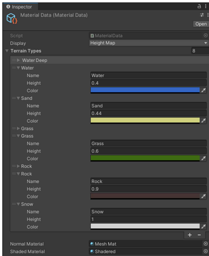
Obrázek 121 - Material Data
