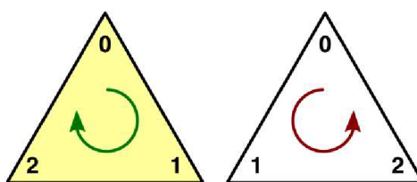
Obrázek 55 - Vrcholy Polygonu
