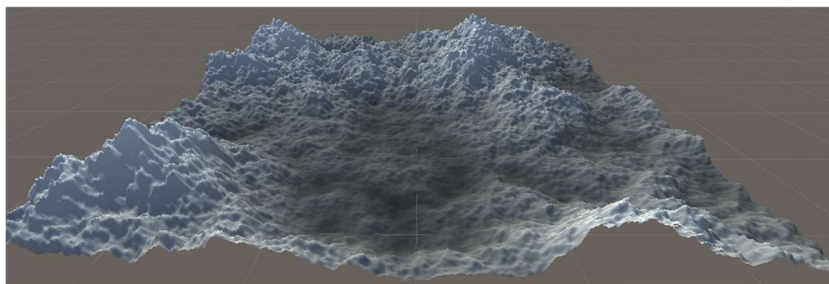
Obrázek 101 - Příklad terénu 1
