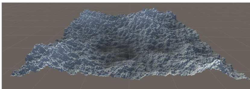
Obrázek 102 - Příklad terénu 2
