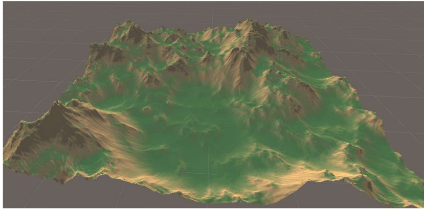
Obrázek 115 - Shaded terén
