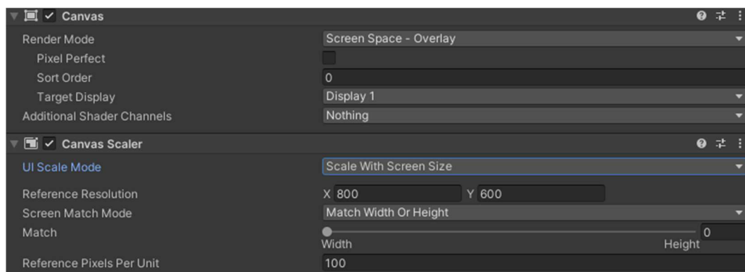
Obrázek 68 - Canvas
