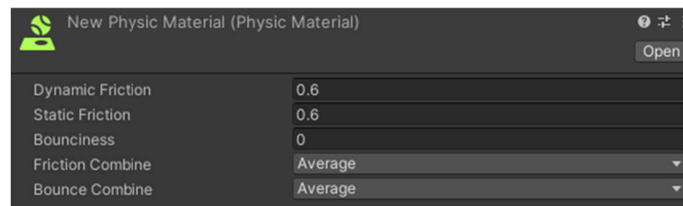
Obrázek 82 - Physic Material
