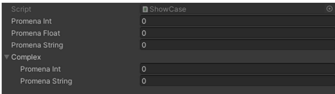
Obrázek 23 - Zobrazení serializaci
