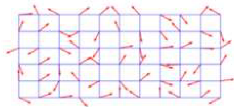
Obrázek 4 - Noise | Grid
