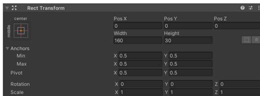
Obrázek 70 - Rect Transform
