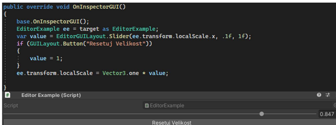
Obrázek 42 - Tlačítka v inspektoru
