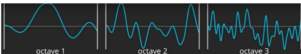
Obrázek 9 - Oktávy (vytvořeno pomocí: http://www.maxmcarter.com/sinewave/sinegen.html )
