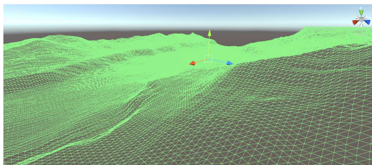
Obrázek 80 - Kolize Collider
