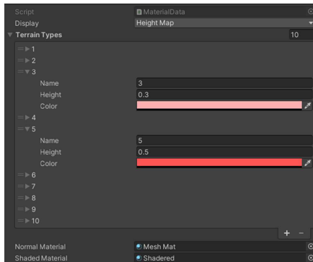
Obrázek 45 - ScriptableObject editor
