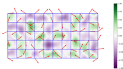
Obrázek 6 - Noise | Inerpolation
