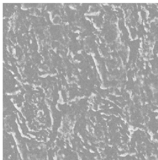
Obrázek 64 - Textura | Metalic
