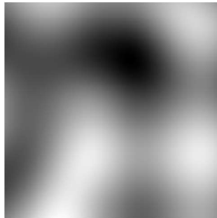
Obrázek 89 - Perlin Noise
