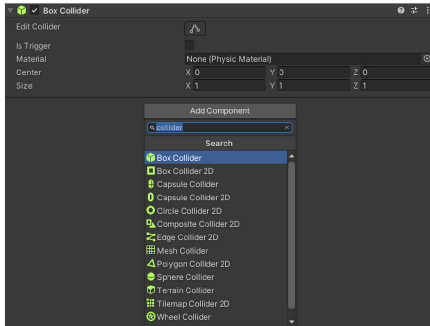
Obrázek 77 - Existující Collidery
