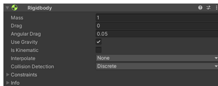
Obrázek 81 - Rigidbody
