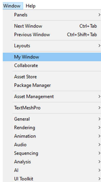
Obrázek 48 - MenuItem tlačítko
