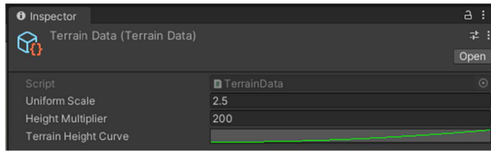
Obrázek 119 - Terrain Data
