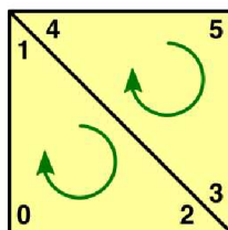
Obrázek 56 - Vrcholy Quad
