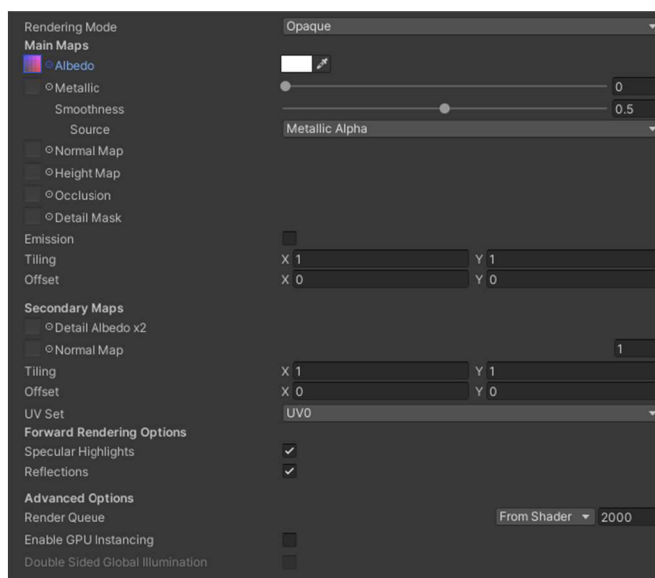
Obrázek 62 - Material
