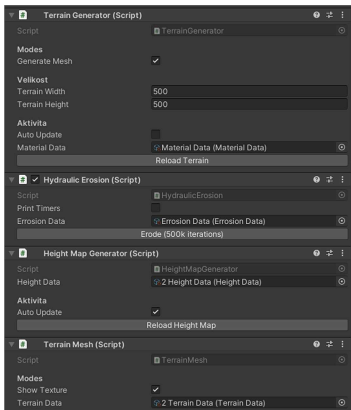
Obrázek 123 - MonoBehaviourura
