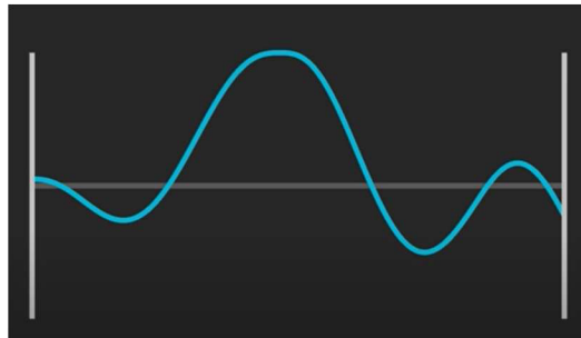
Obrázek 1 - Změny výšky (vytvořeno pomocí: http://www.maxncarter.com/sinewave/sinegen.html )
