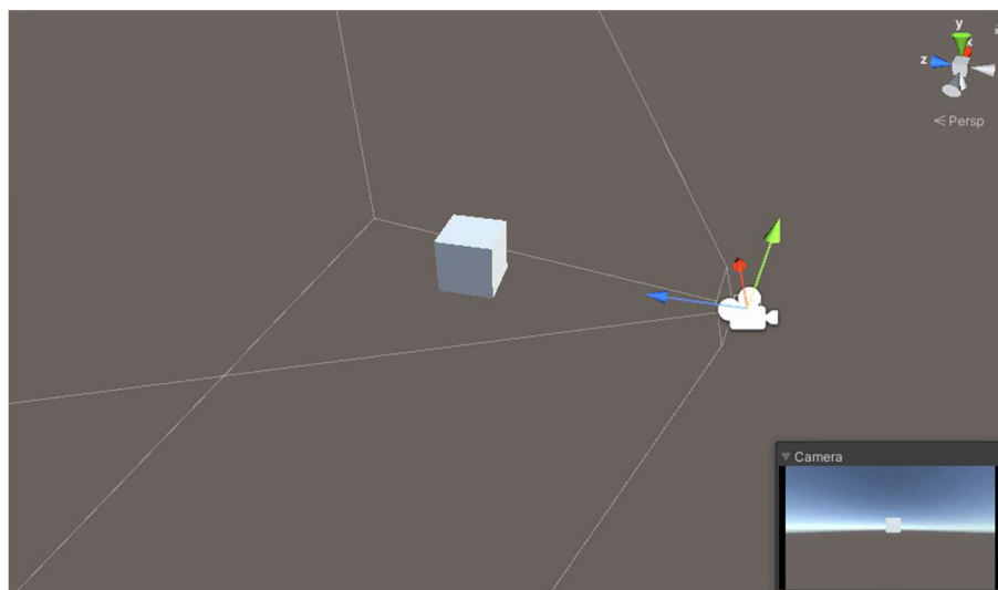
Obrázek 59 - Kužel kamery
