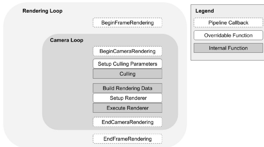
Obrázek 51- Redner loop
