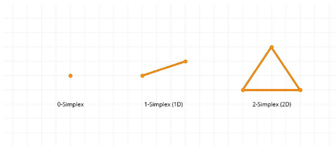
Obr. 4.8: Typy simplexov.
