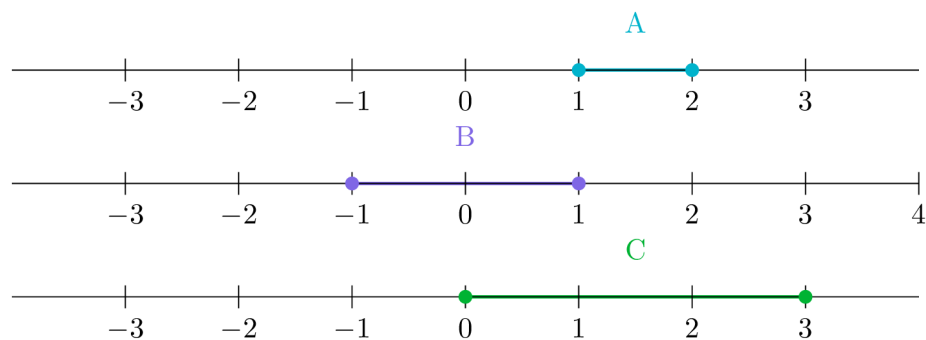
Obr. 4.7: Kolíže regiónov
