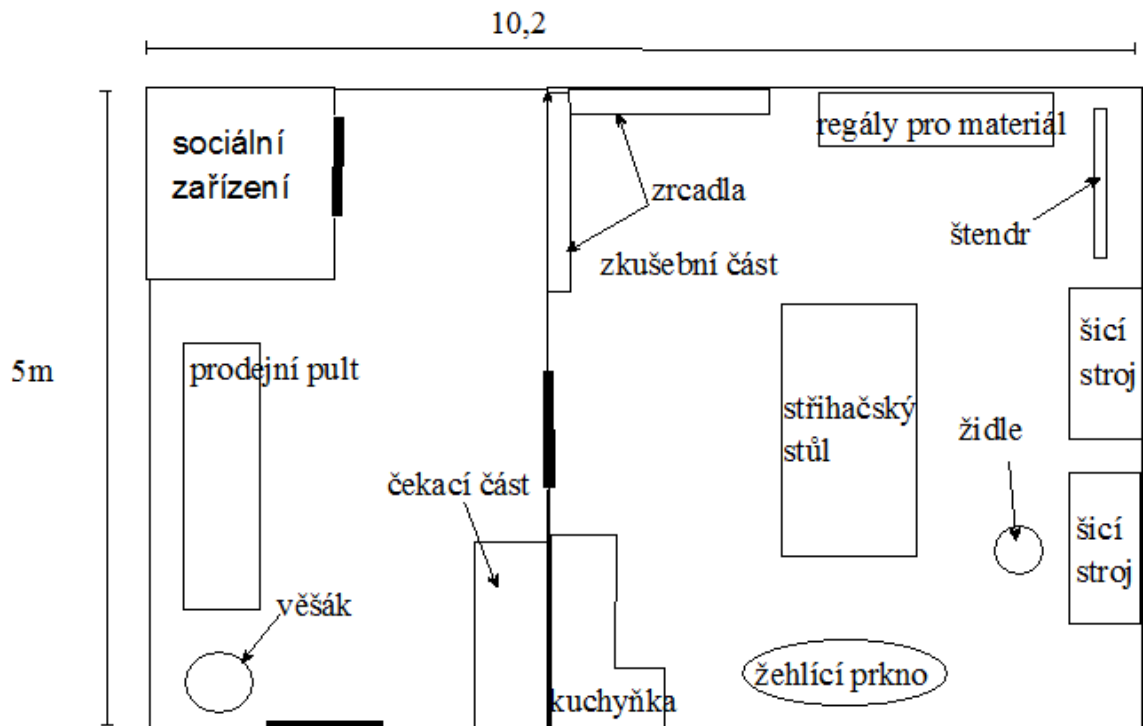
Obrázek 7 Půdorys krejčovského salónu
