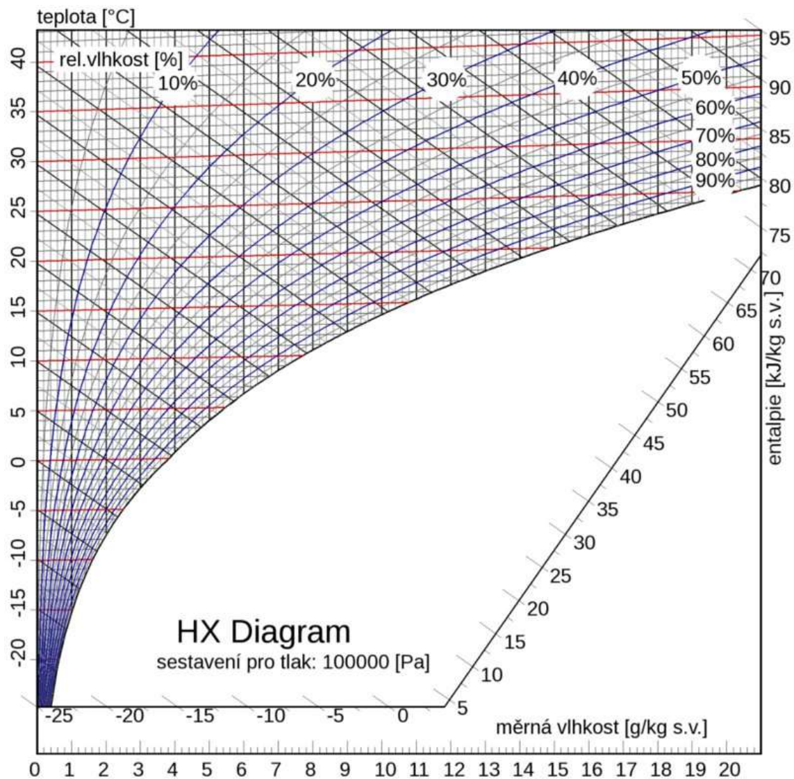
Obrázek 7.- HX Diagram
