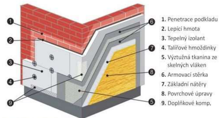
Obrázek 20.- Skladba kontaktního zateplovacího systému
