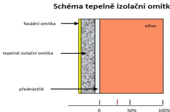
Obrázek 19.- Tepelně izolační omítka
