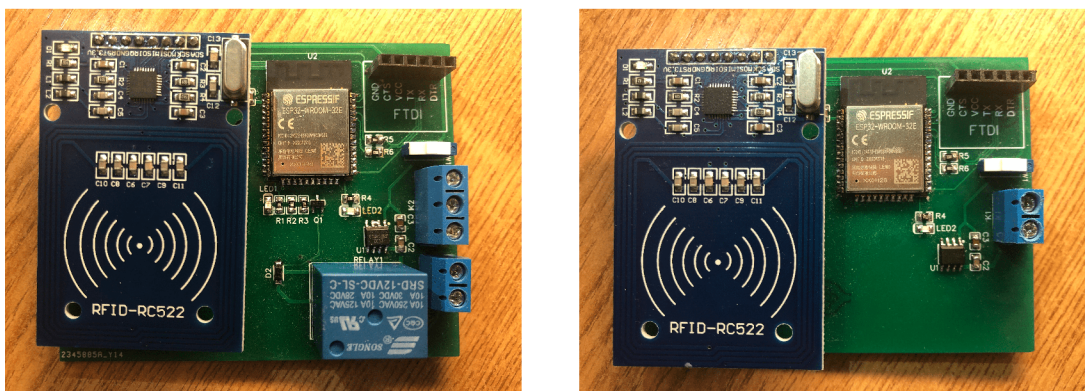
(a) Osazená deska zámkových modulů
