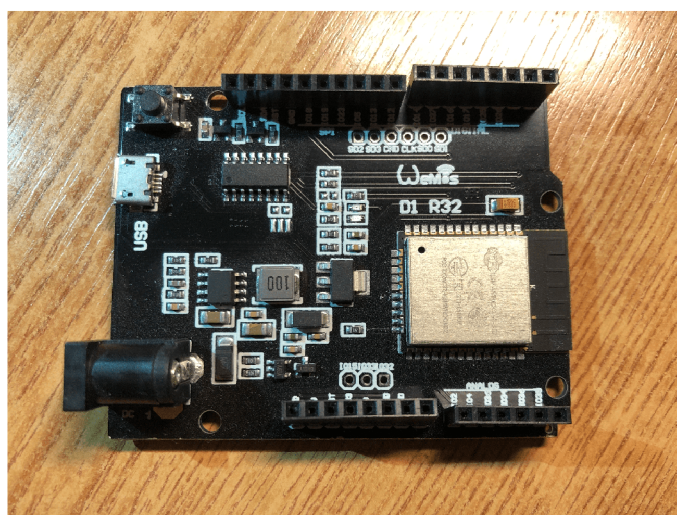
Obrázek 3.3: Vývojová deska Wemos D1 R32
