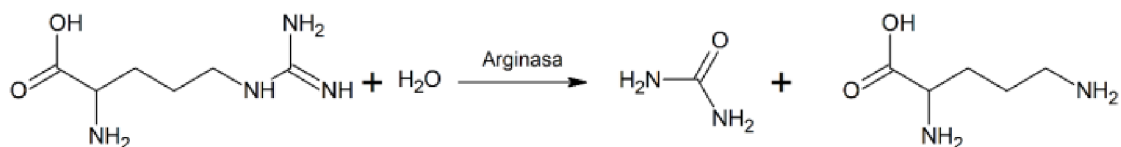
Obrázek 2 Reakce katalyzovaná arginásou
