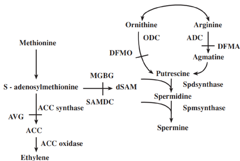
Obrázek 1 Biosyntéza polyaminů
