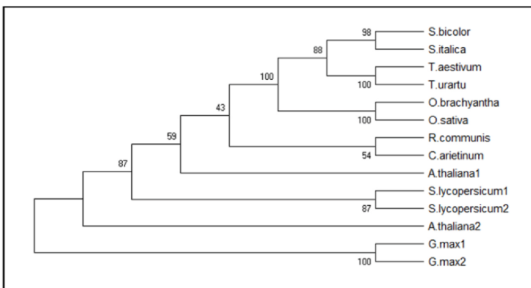
Obrázek 4 Fylogenetický strom
