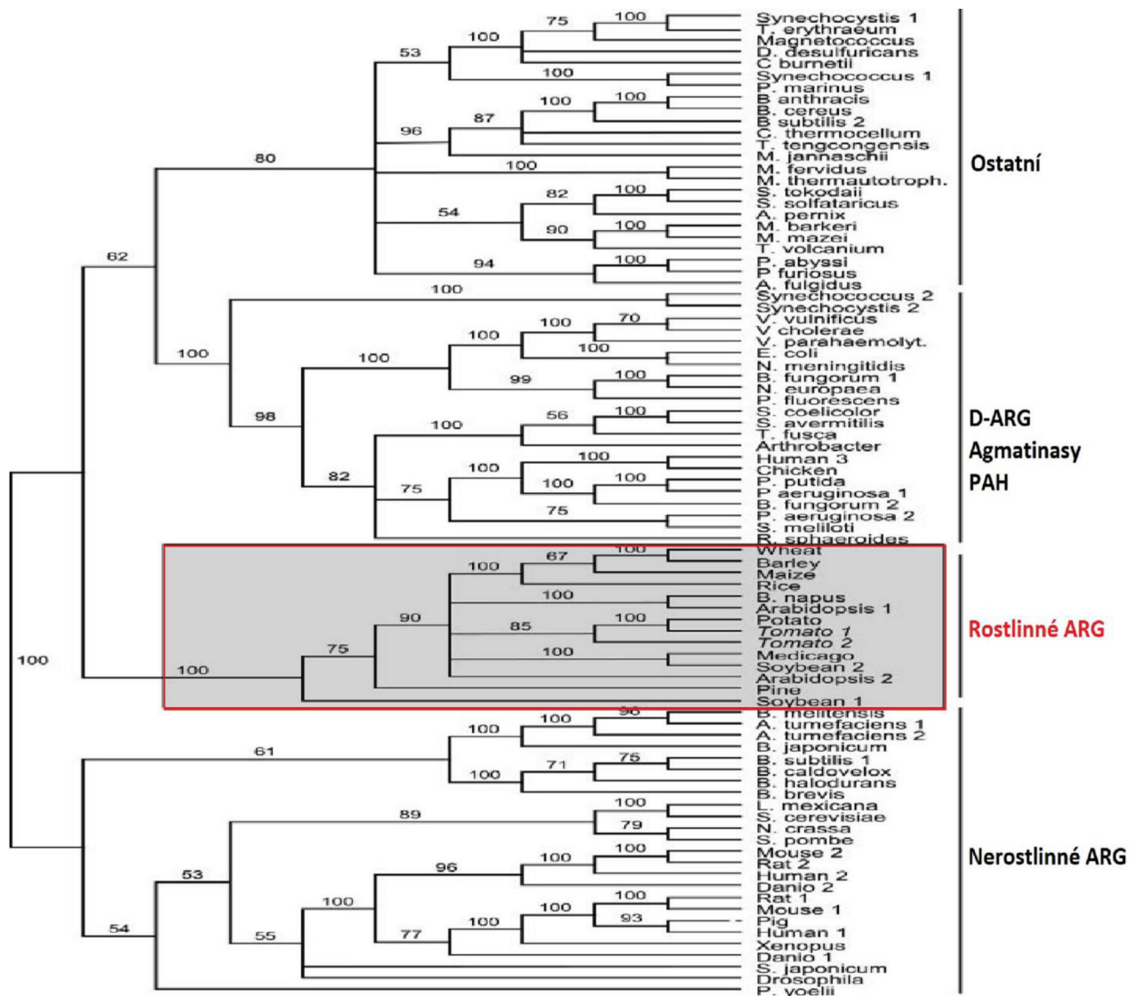
Obrázek 3 Fylogenetický strom 85 amidinohydrolas, PAH – prokavaminátamidinohydrolasy. (Přepřacováno podle Chen et al. , 2004)
