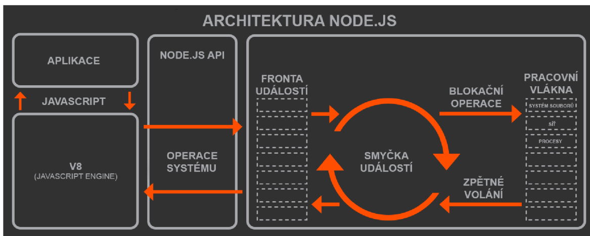
Obrázek 8: Architektura Node.js (22)
