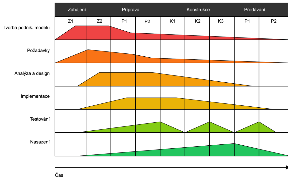
Obrázek 3: RUP model (4)
