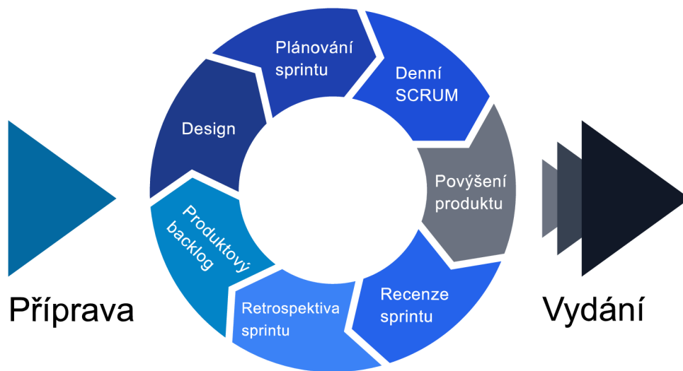
Obrázek 4: SCRUM způsob (5)
