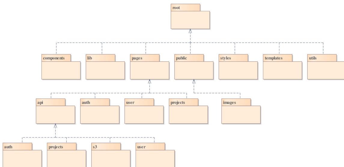
Obrázek 16: Struktura projektu
