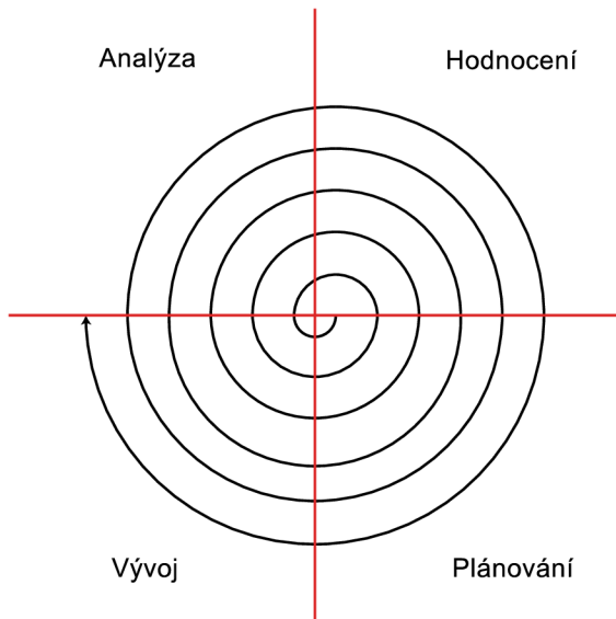
Obrázek 2: Spirálový model (3)
