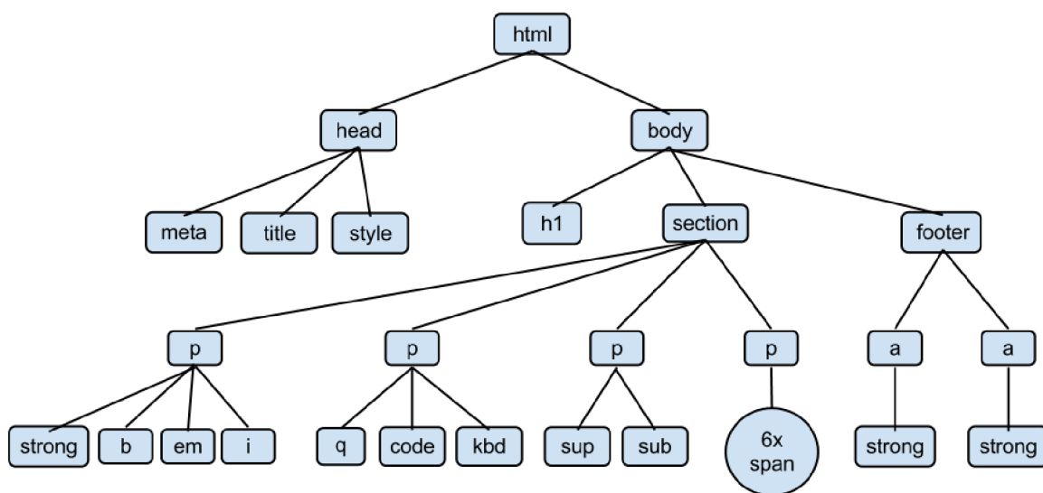
Obrázek 5: DOM strom (9)
