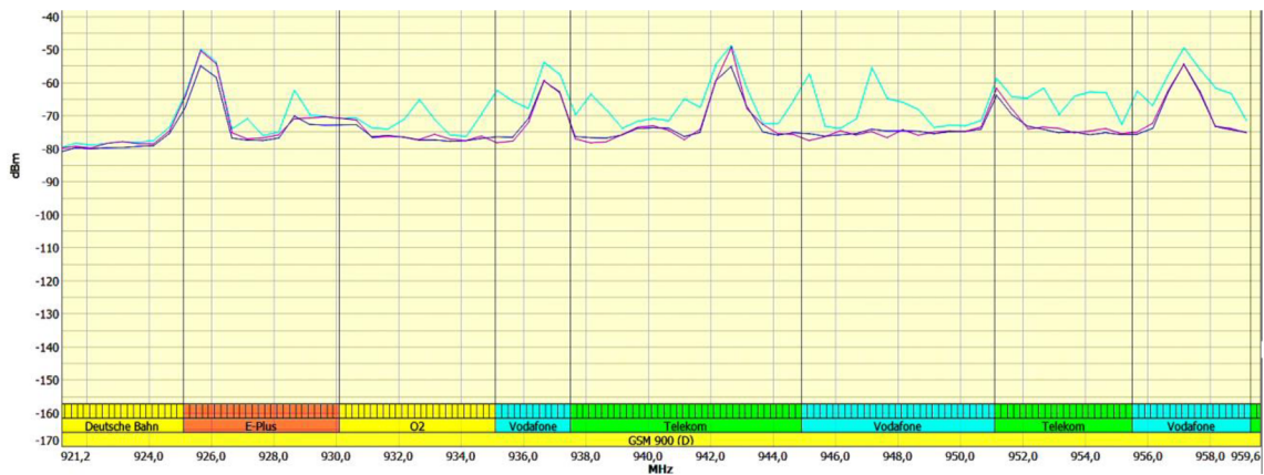
Obrázek 10 - Byt - 900 MHz
