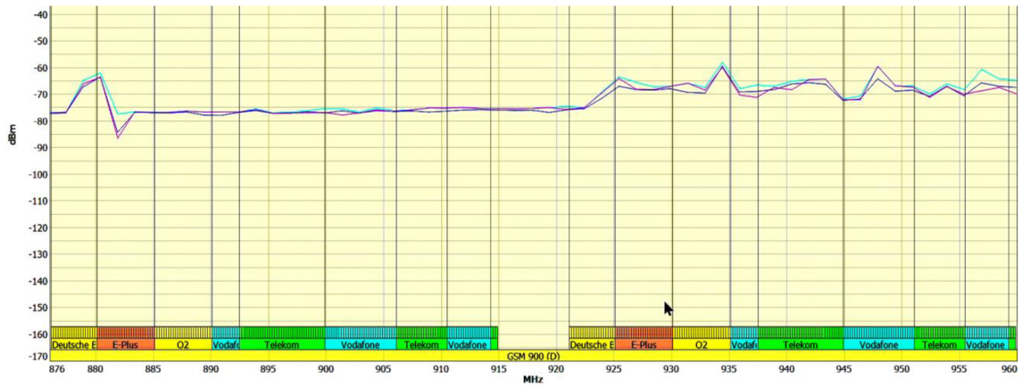
Obrázek 11 - Koleje - 900 MHz
