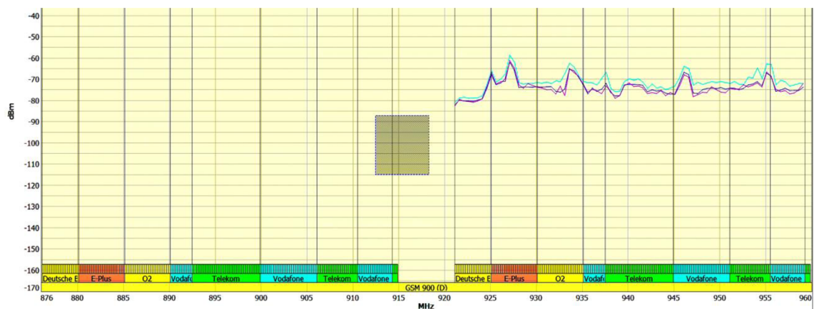
Obrázek 16 - Obsazená kóje - 900 MHz
