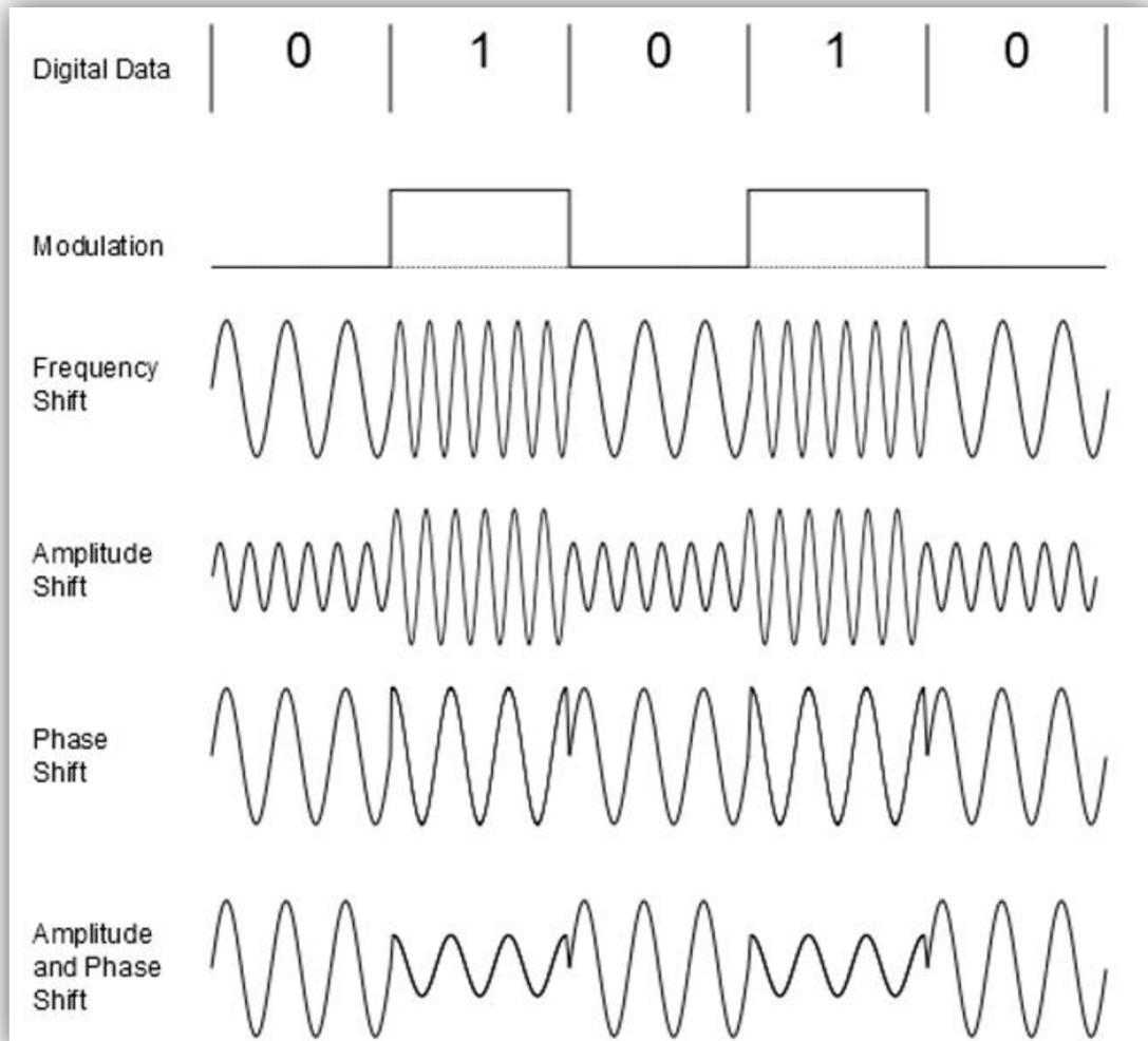
Obrázek 6 - Kvadrurní amplitudová modulace (Anon 2023)
