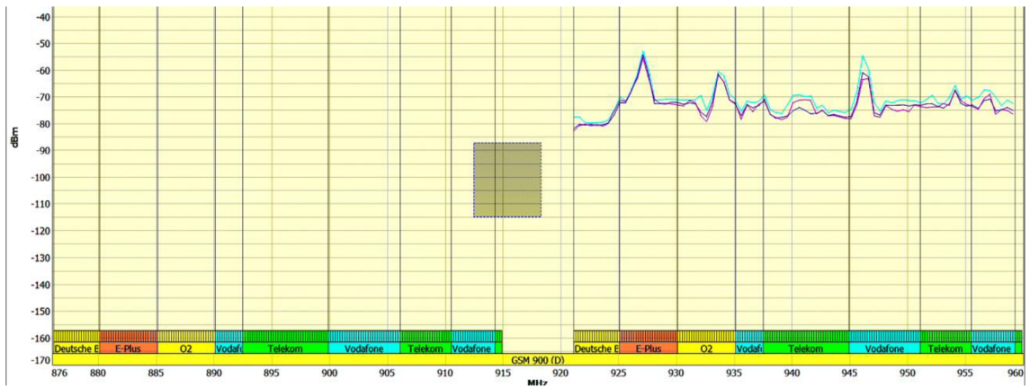
Obrázek 13 - Meziprostor - 900 MHz
