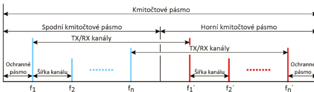
Obrázek 2 - Uspořádání kmitočtového pásma (Anon 2012)
