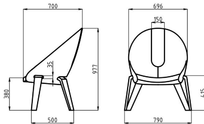
Obr. 4-6 Varianta I – základní rozměry
