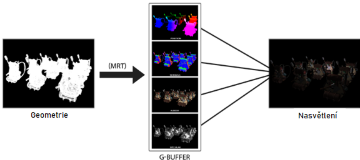
Obrázek 4 Znáznornění Deferred rendering přístupu (De Vries, 2024)
